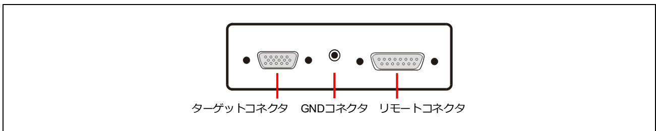
図2.3 FP6 ホストインタフェース面
