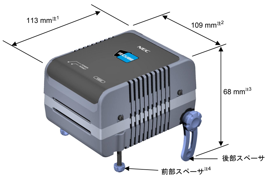
図1 - 1 外形寸法
