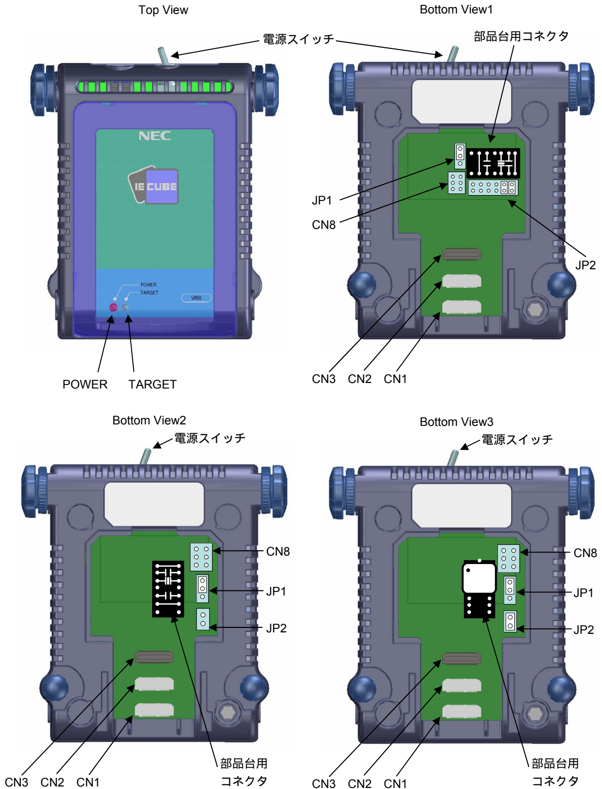
図2 - 1 QB-V850ESSX2の各部の名称
