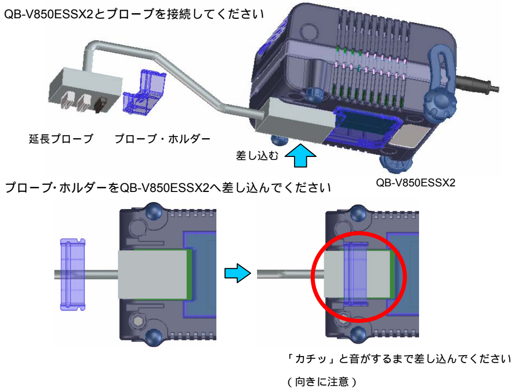
図2 - 14 プローブ・ホルダーの使用方法
