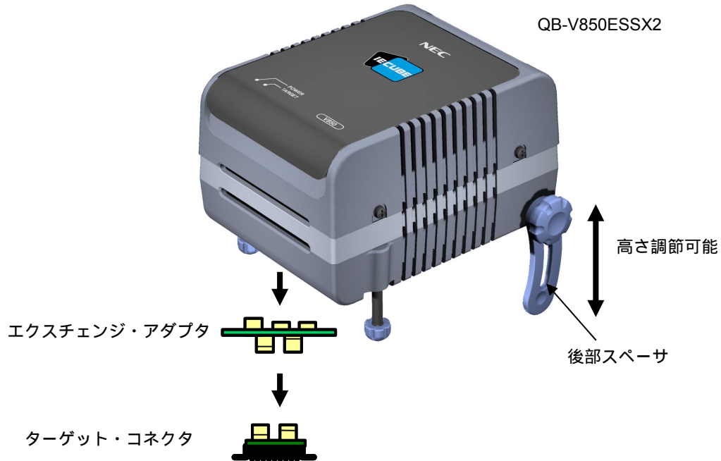
図2 - 13 延長プローブを使用しない場合の接続
