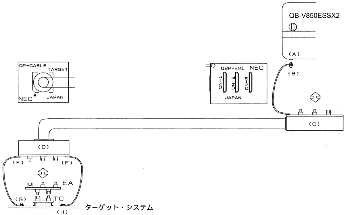
図2 - 15 GND線
