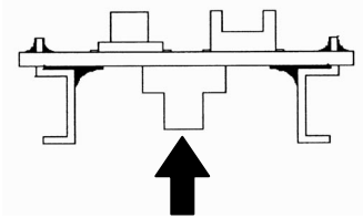
図2 - 11 TC突起図
