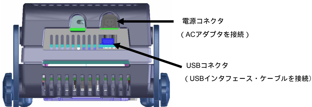
図2 - 18 コネクタ位置
