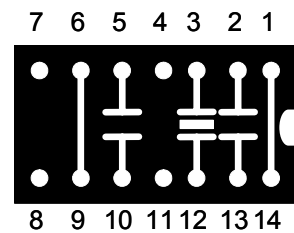
図2 - 5 部品台設定
