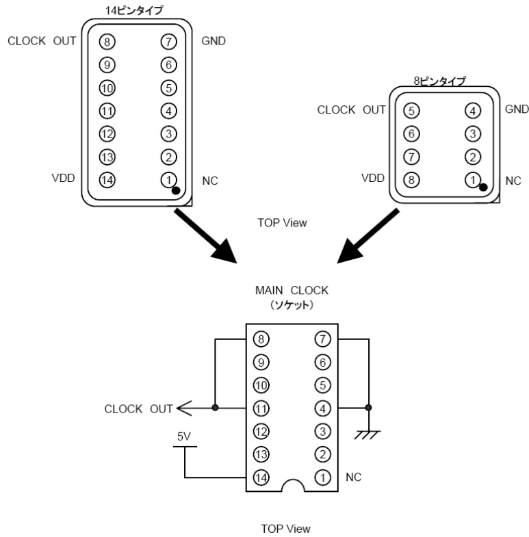
図2 - 3 MAIN CLOCKの実装方法
