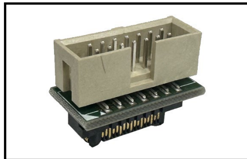
図 1 RTE0T00020KCA30000J の外観
