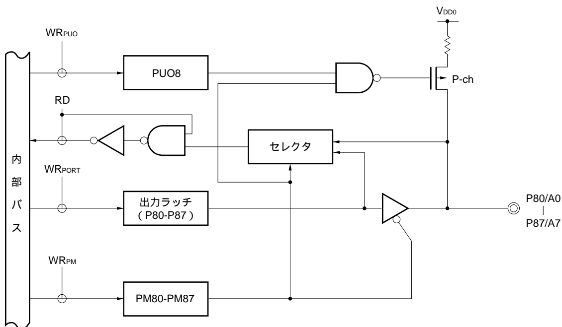
図6-17 P80-P87のブロック図
