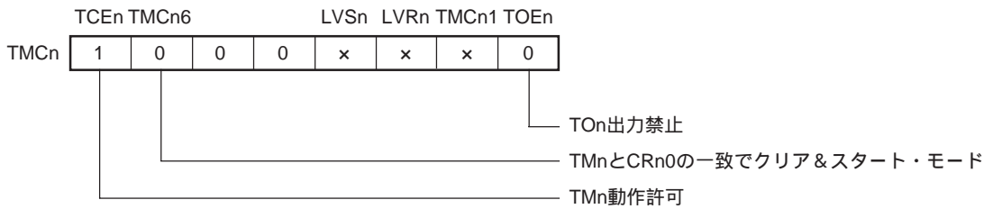
図10 - 10 外部イベント・カウンタ動作時の8ビット・タイマ・モード・コントロール・レジスタの設定内容
