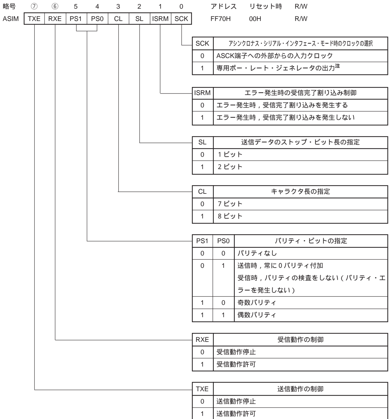
図20 - 4 アシクロナス・シリアル・インタフェース・モード・レジスタのフォーマット
