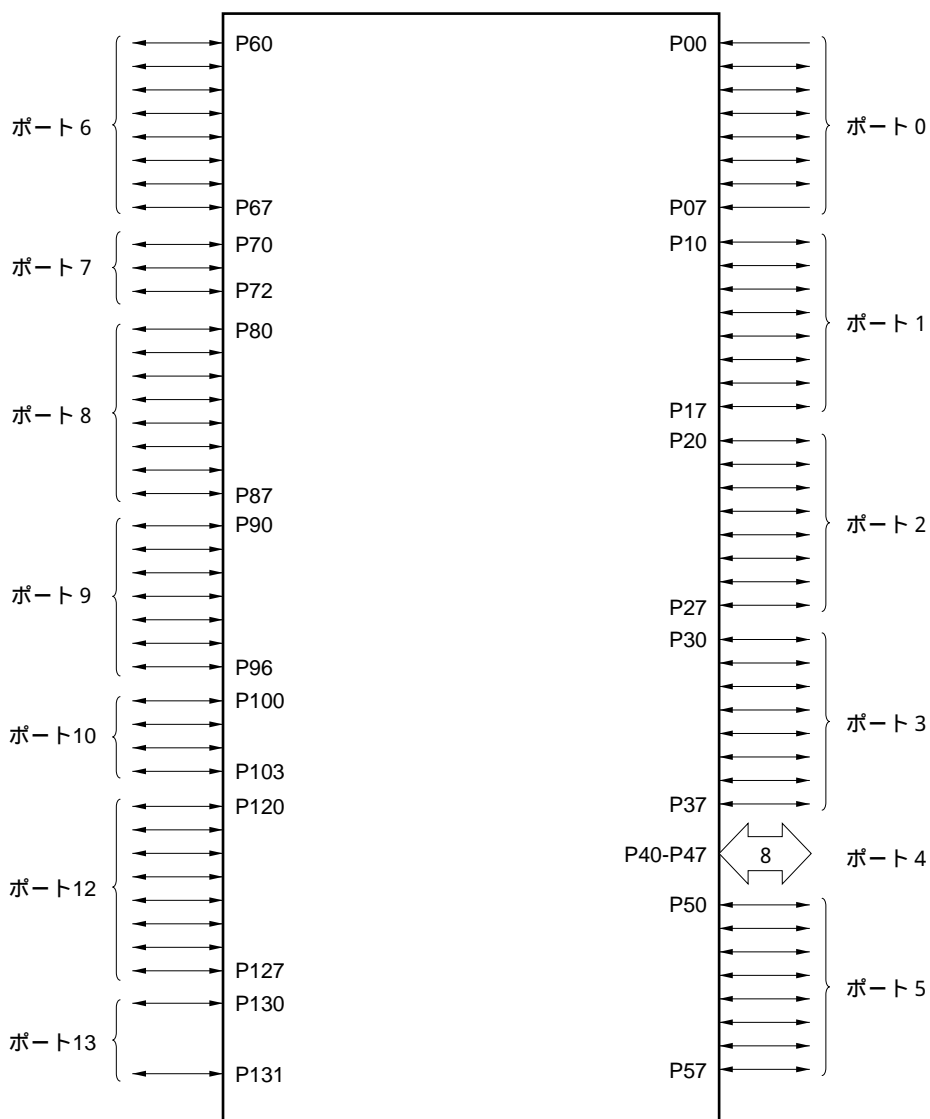
図6-1 ポートの種類
