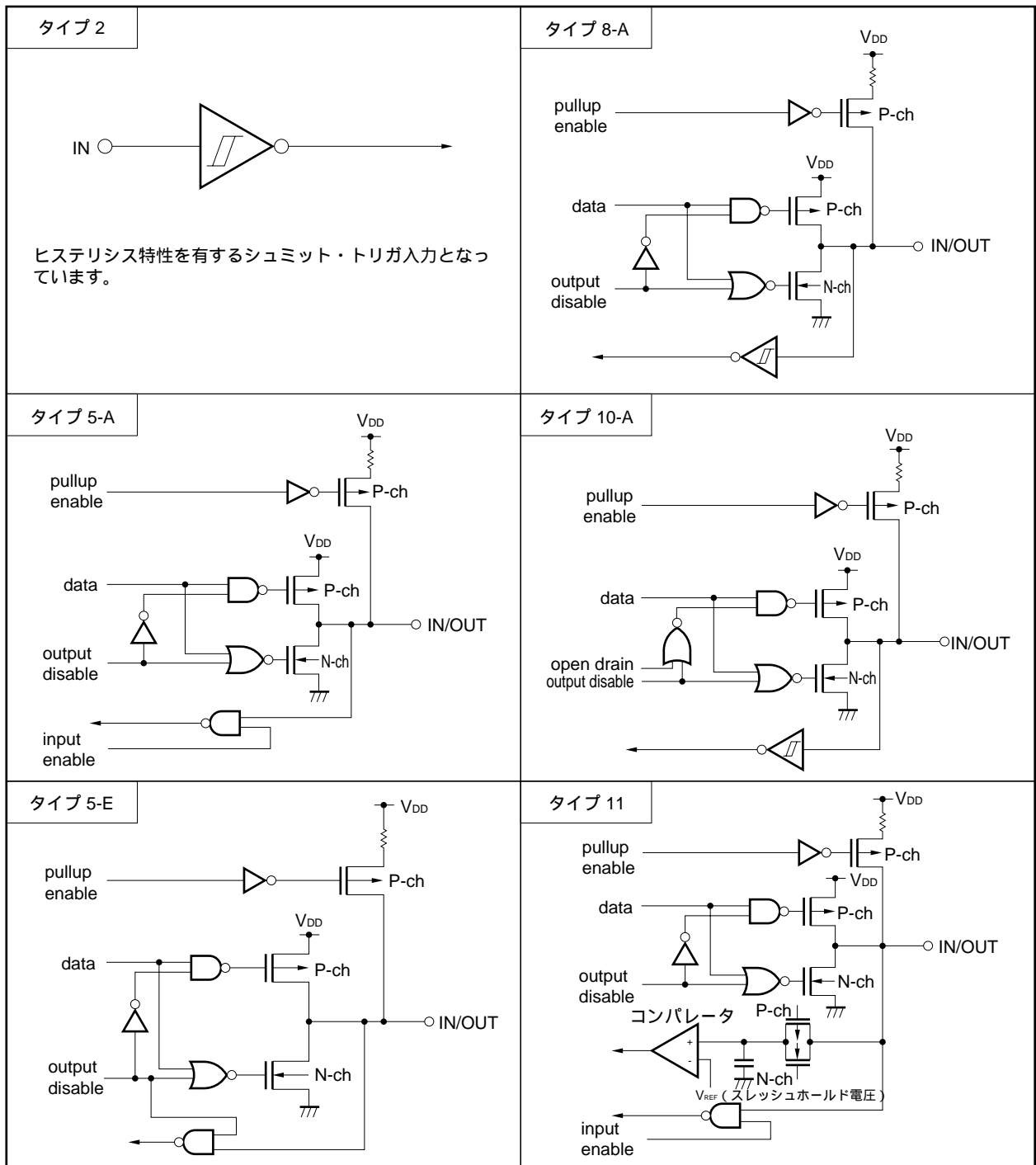
図26 - 1 端子の入出力回路一覧 (1/2)
