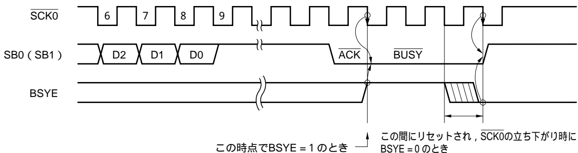
図17-25 BSYEの動作
