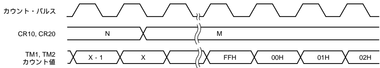
図9 - 16 タイマ・カウント動作中のコンペア・レジスタの変更後のタイミング
