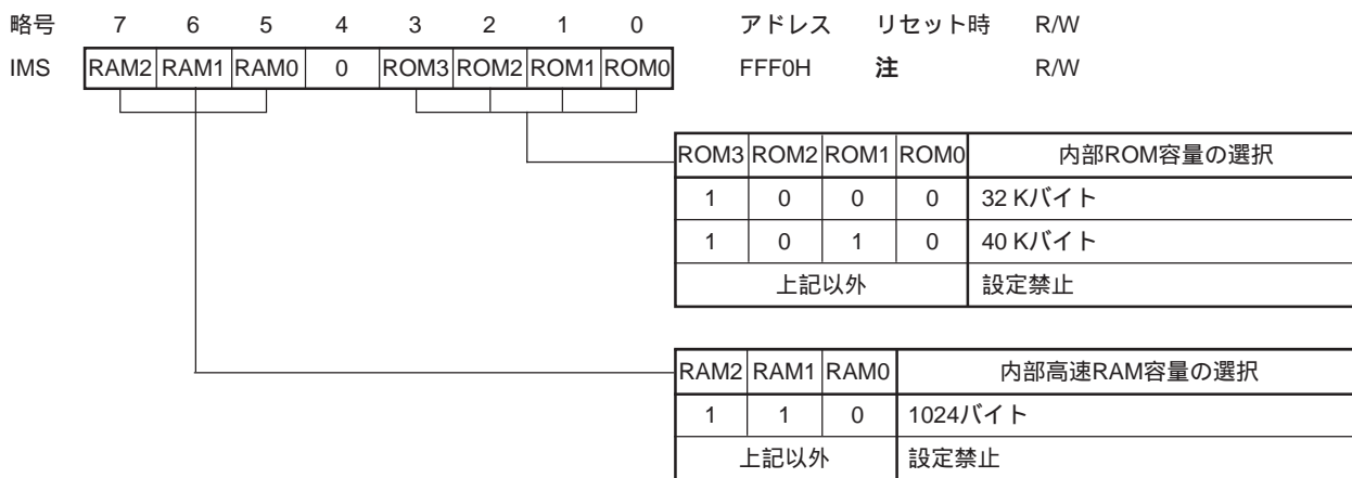
図23 - 3 メモリ・サイズ切り替えレジスタのフォーマット
