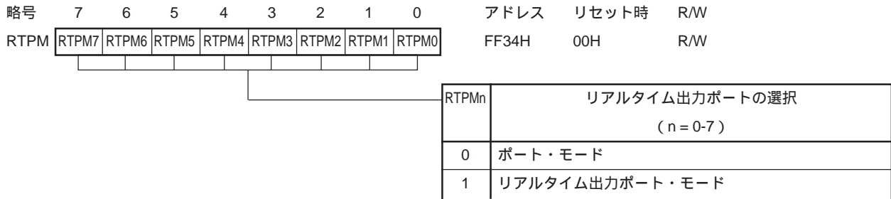
図21 - 4 リアルタイム出力ポート・モード・レジスタのフォーマット
