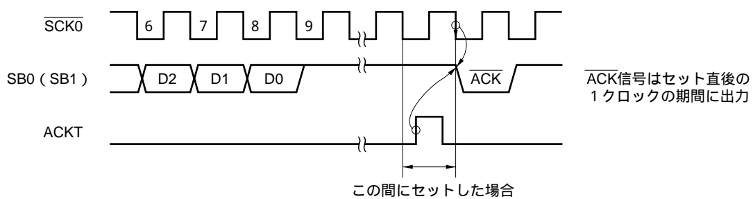
図17 - 22 ACKTの動作
