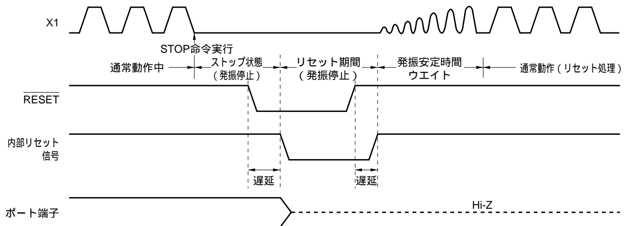
図25 - 4 STOPモード中のRESET 入力によるリセット・タイミング
