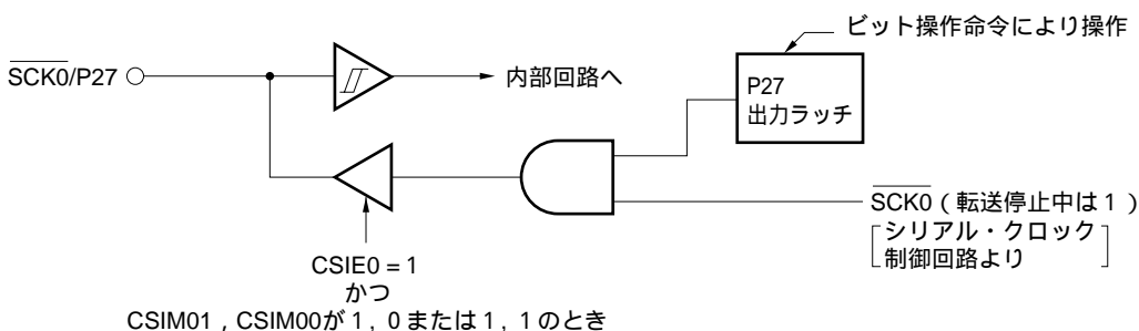
図17-34 SCK0/P27端子の構成
