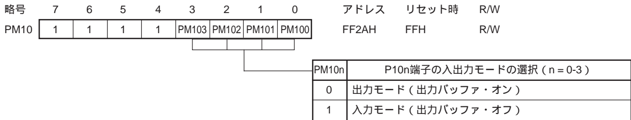
図10-7 ポート・モード・レジスタ10のフォーマット
