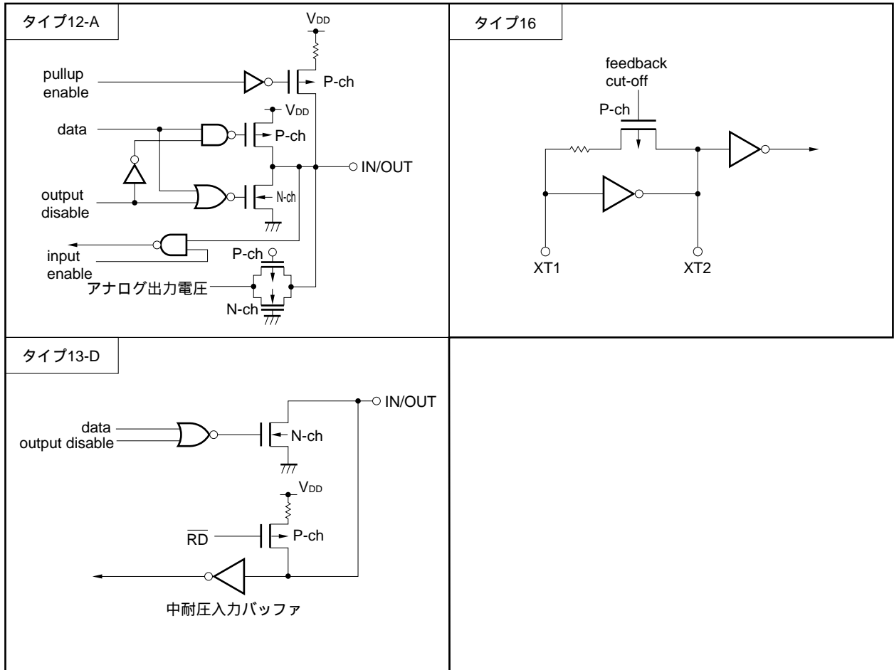
図26 - 2 端子の入出力回路一覧 (2/2)
