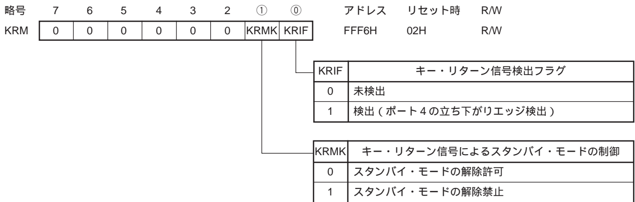
図6-27 キー・リターン・モード・レジスタのフォーマット
