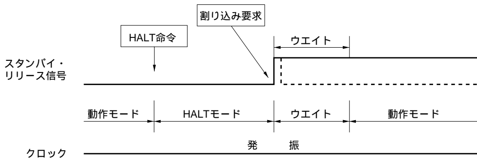
図24 - 2 HALTモードの割り込み要求発生による解除
