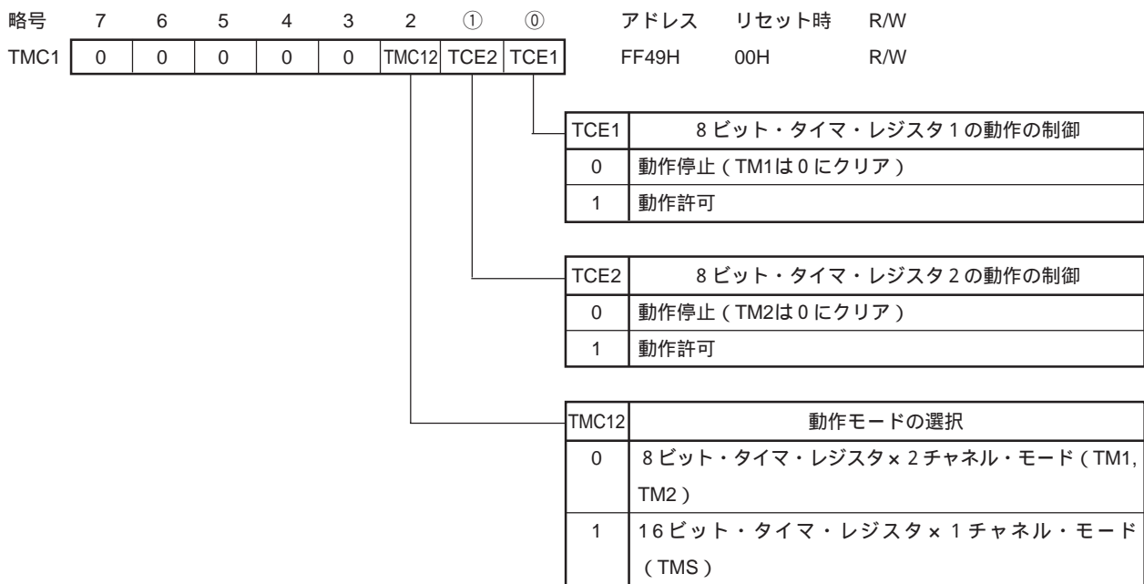
図9 - 5 8ビット・タイマ・モード・コントロール・レジスタ1のフォーマット
