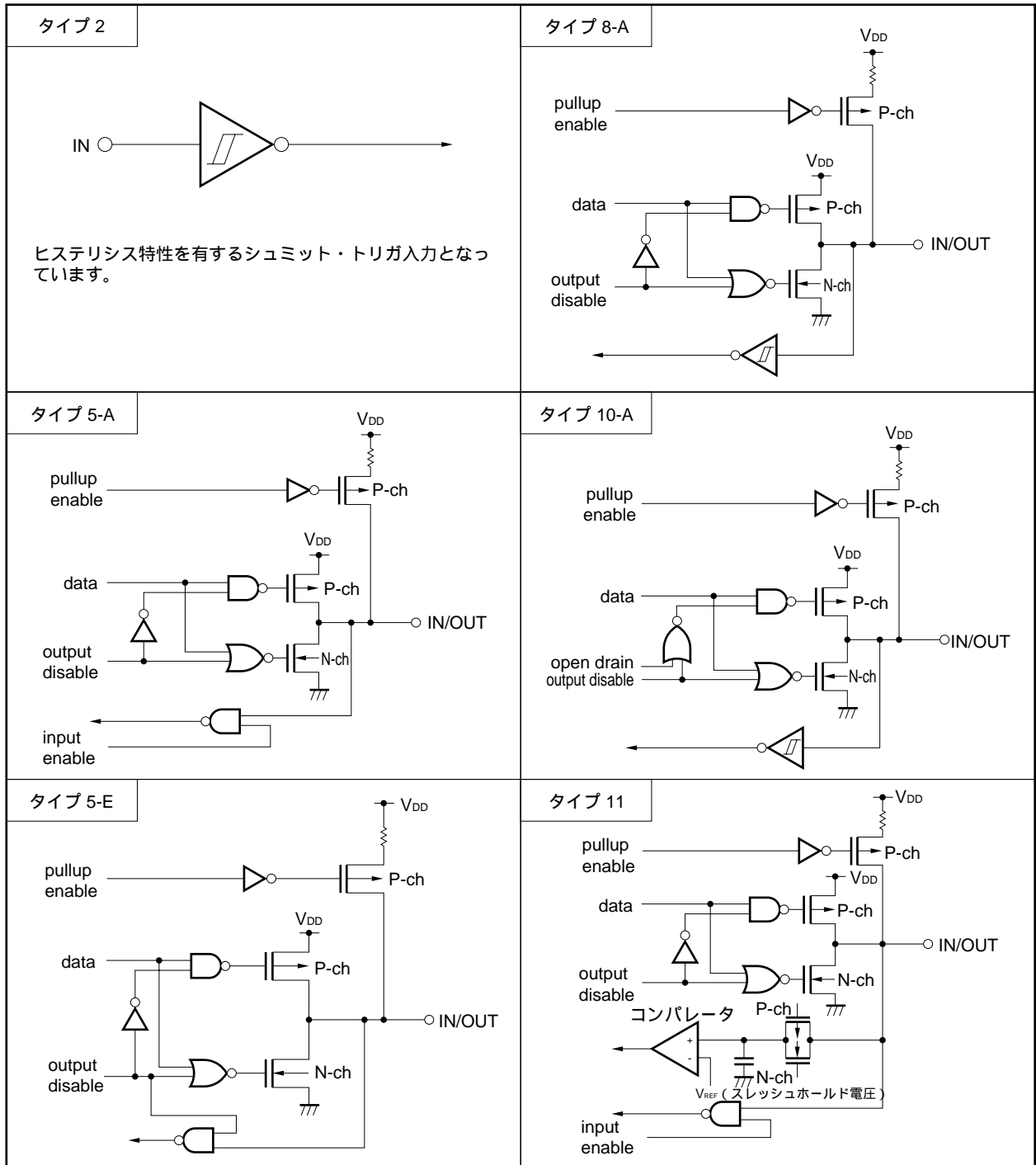
図26 - 2 端子の入出力回路一覧 (1/2)
