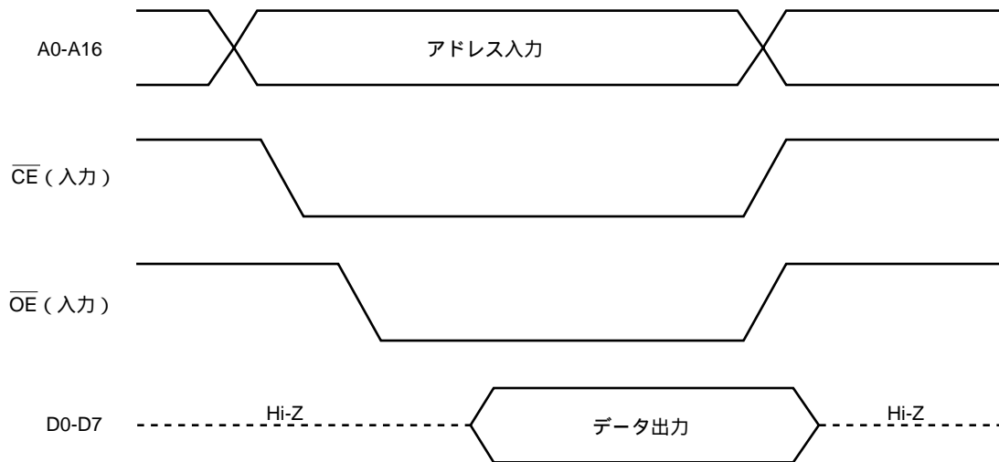
図26-9 PROMの読み出しタイミング
