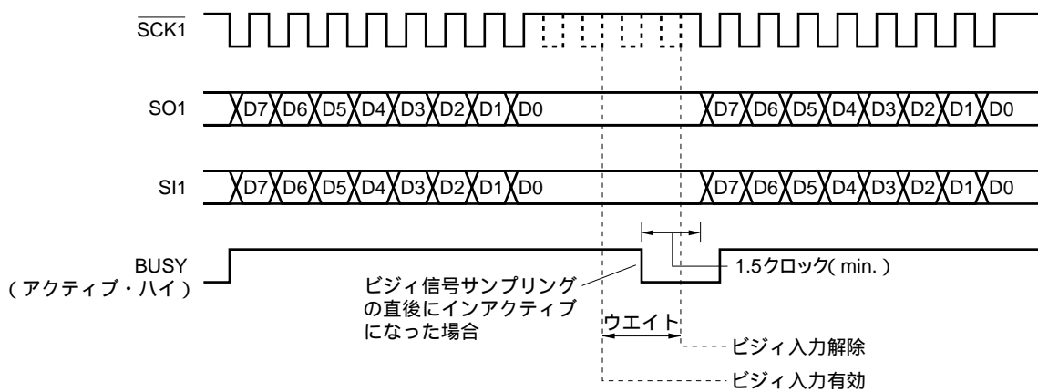
図19 - 20 ビジィ信号とウエイトの解除 (BUSY0 = 0のとき)
