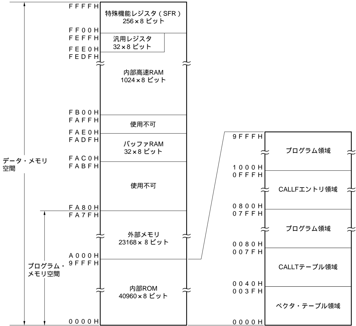
図5 - 2 メモリ・マップ (μPD78075B, 78075BY)
