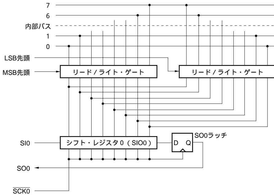
図17 - 9 転送ビット順切り替え回路
