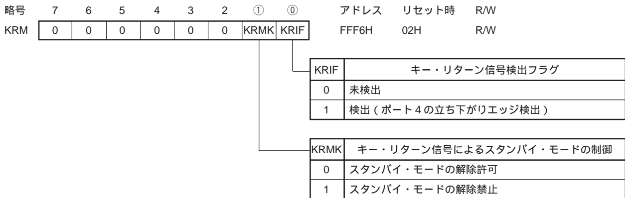
図22-21 キー・リターン・モード・レジスタのフォーマット
