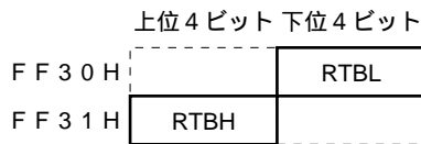
図21 - 2 リアルタイム出力バッファ・レジスタの構成
