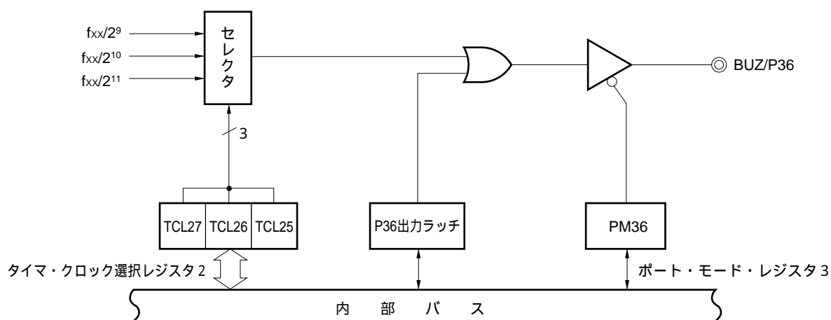
図14 - 1 ブザー出力制御回路のブロック図
