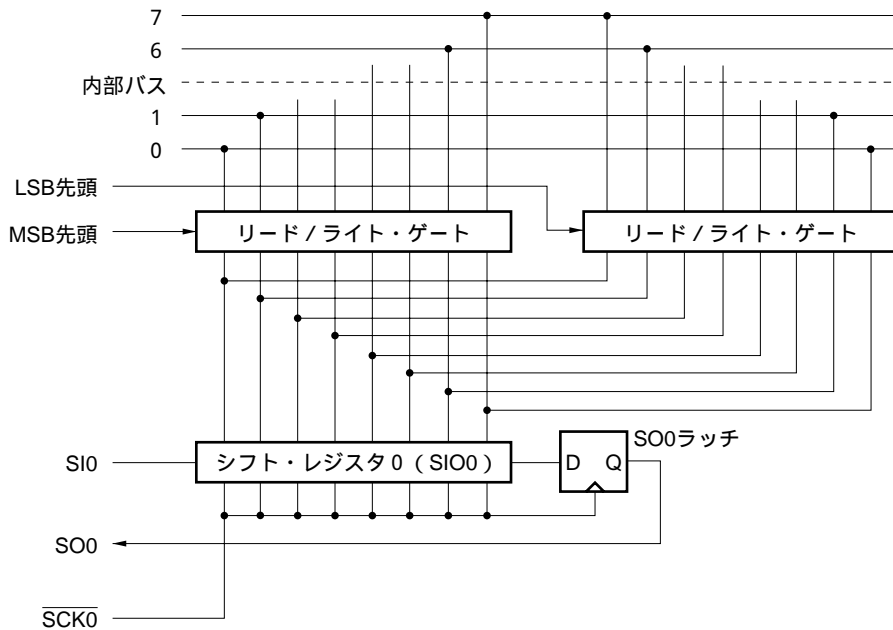
図18 - 9 転送ビット順切り替え回路
