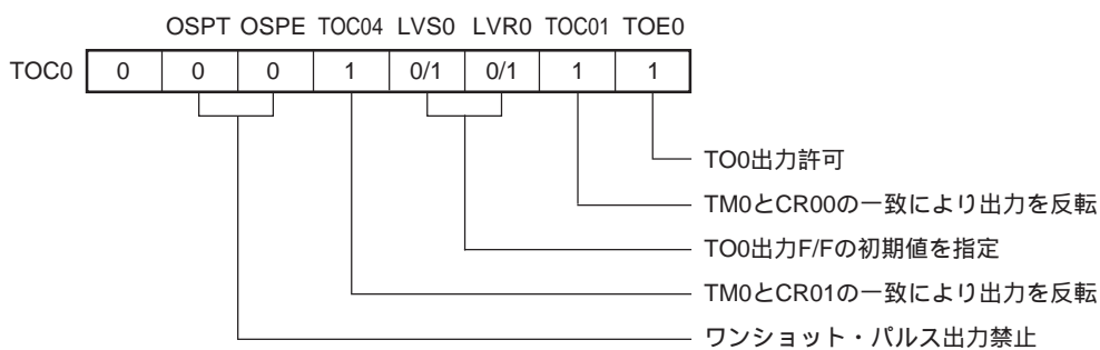
(c) 16ビット・タイマ出力コントロール・レジスタ (TOC0)
