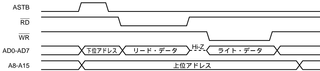
( b ) ウェイトあり ( PW1, PW0 = 0, 1 ) 設定時
