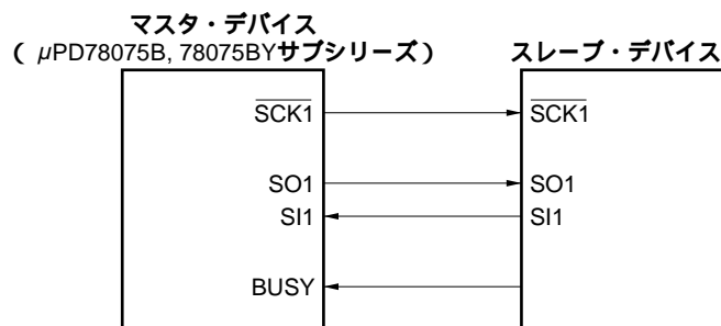
図19 - 18 ビジィ制御オプション使用時のシステム構成
