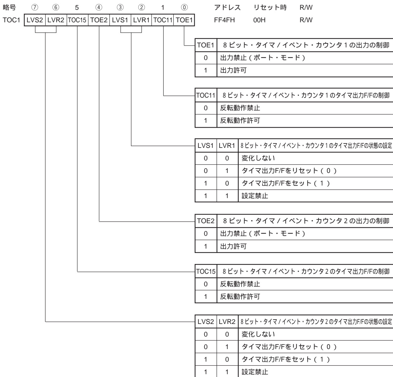
図9-6 8ビット・タイマ出力コントロール・レジスタのフォーマット
