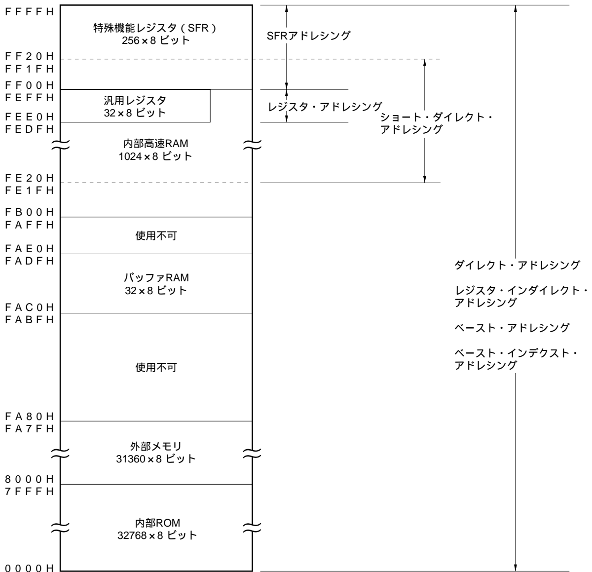
図5 - 3 データ・メモリのアドレッシング（μPD78074B, 78074BY）
