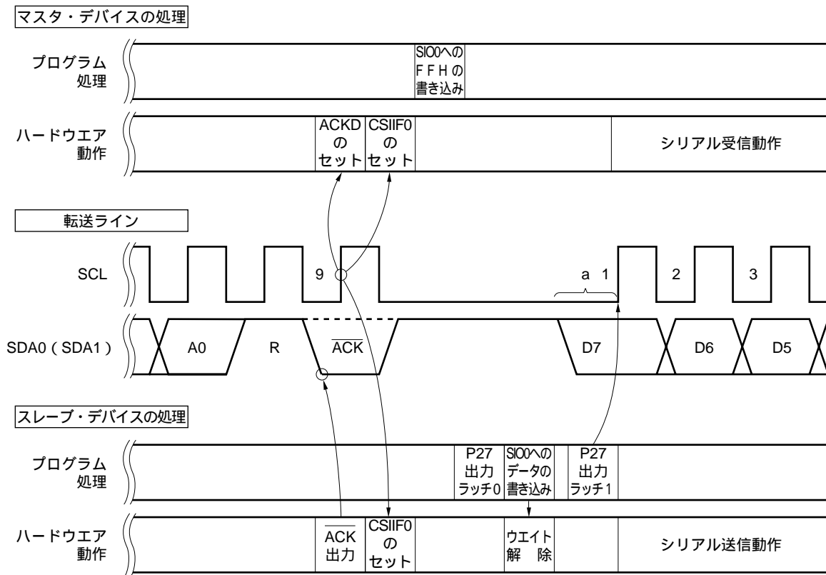
図18-25 スレーブのウェイト解除 (送信時)
