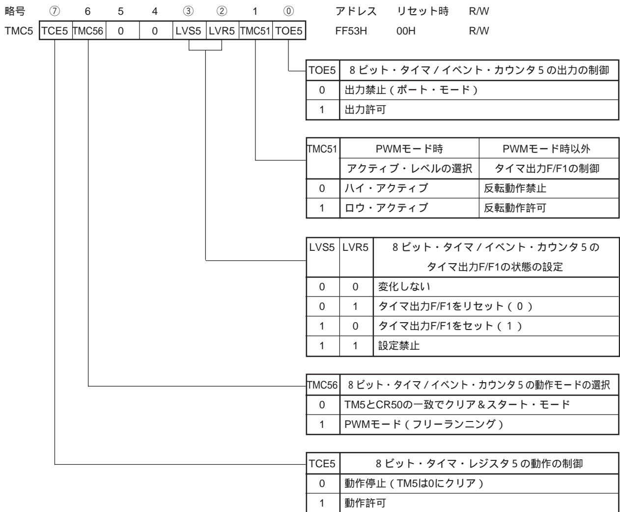
図10-5 8ビット・タイマ・モード・コントロール・レジスタ5のフォーマット
