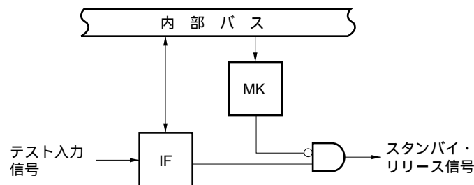
図22 - 18 テスト機能の基本構成
