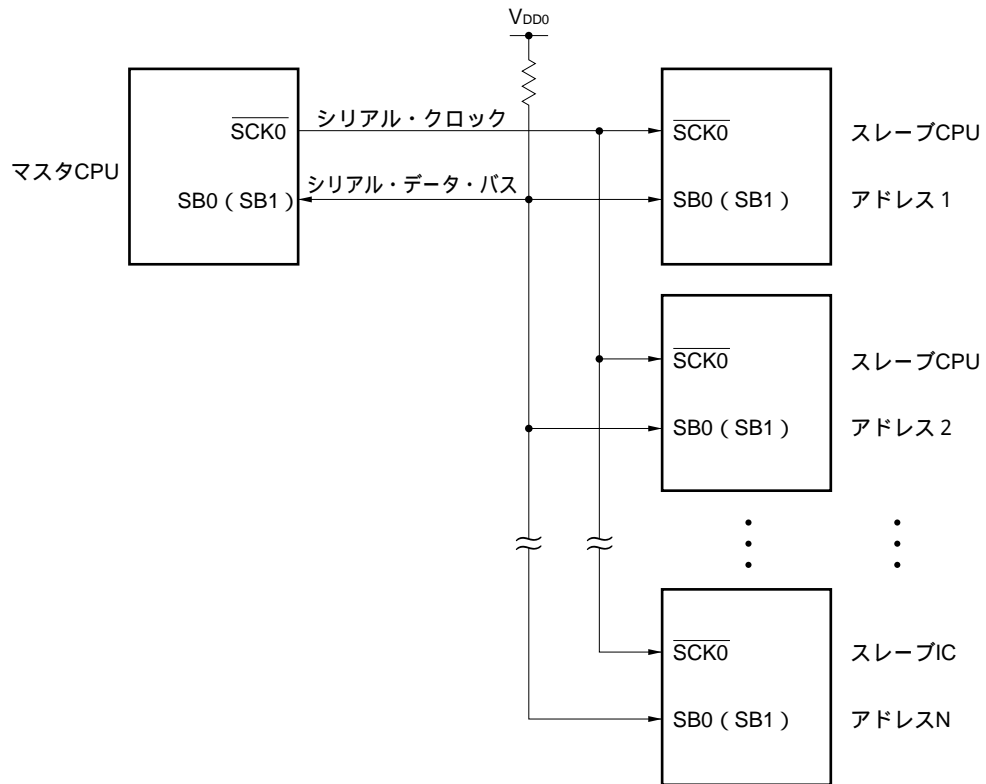
図17 - 10 SBIによるシリアル・バス構成例
