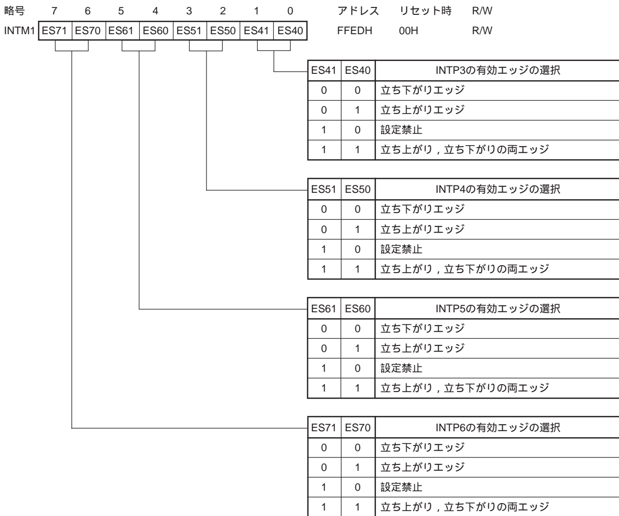
図15 - 4 外部割り込みモード・レジスタ1のフォーマット
