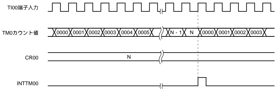
図8 - 28 外部イベント・カウンタ動作のタイミング (立ち上がりエッジ指定時)
