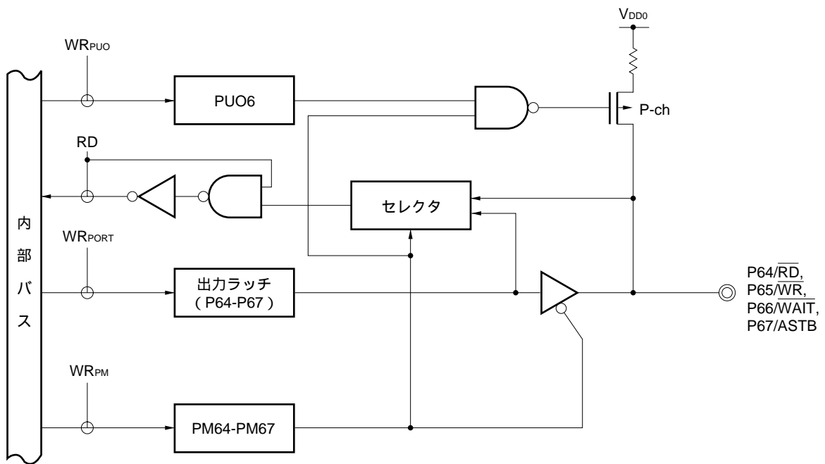
図6 - 14 P64-P67のブロック図
