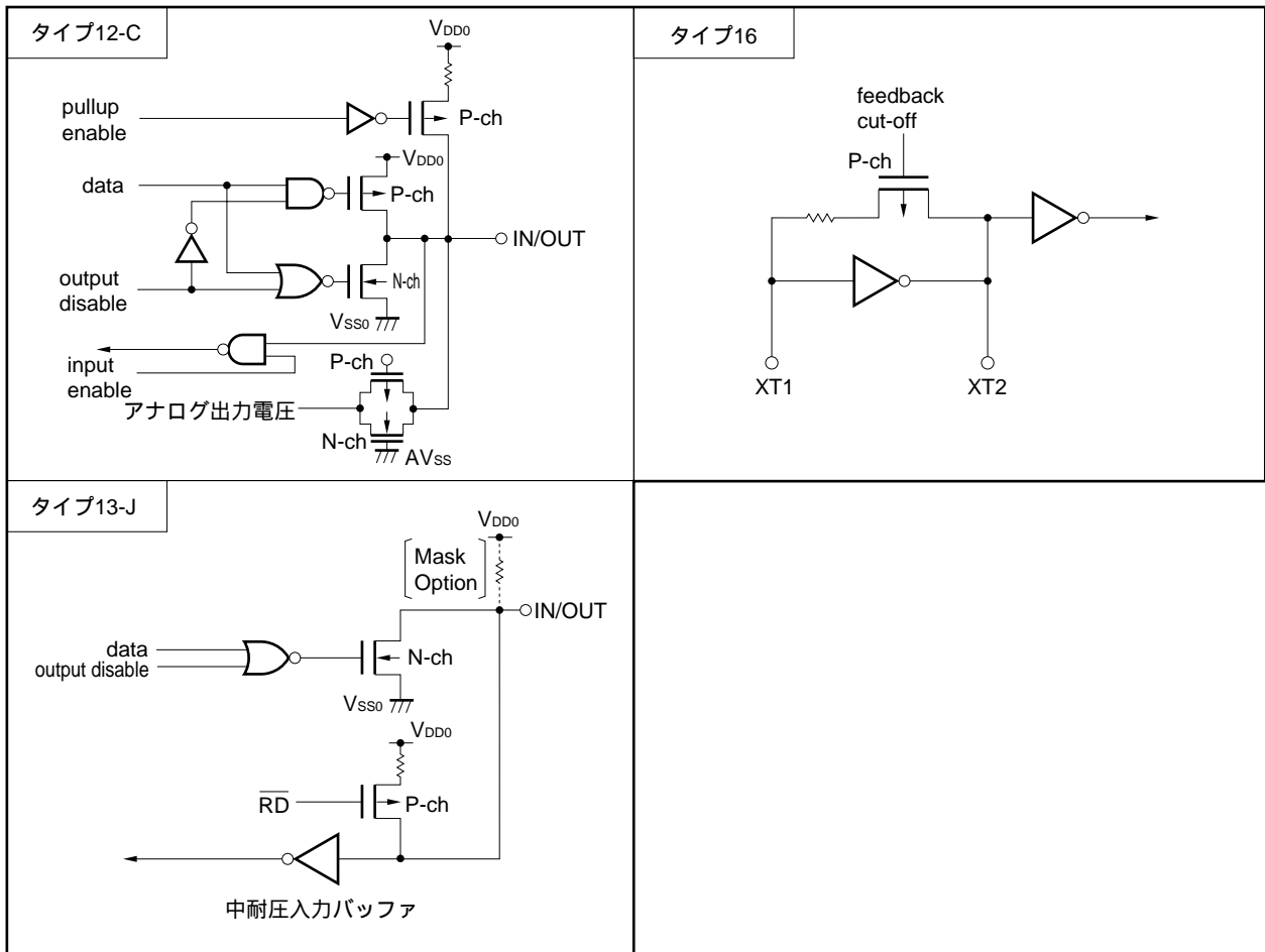
図4-1 端子の入出力回路一覧 (2/2)
