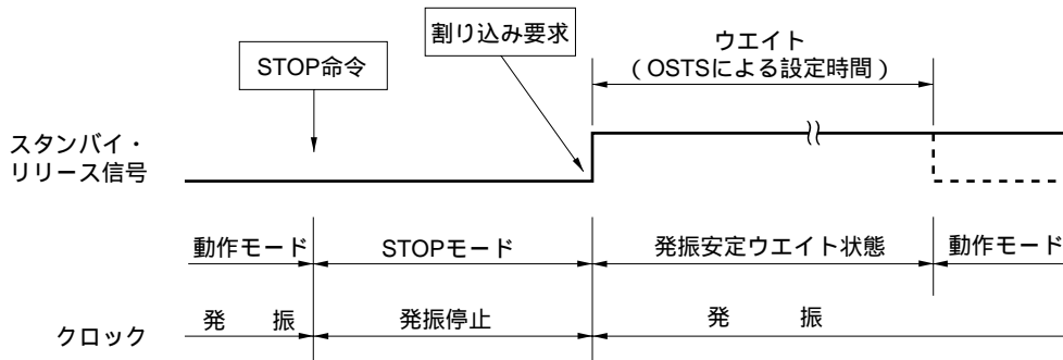
図24 - 4 STOPモードの割り込み要求発生による解除
