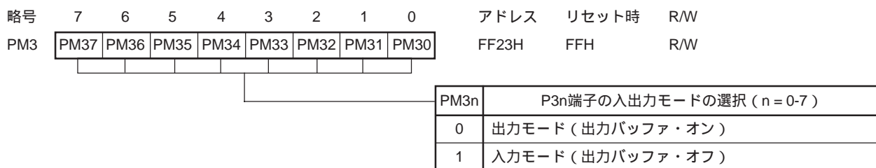
図14 - 3 ポート・モード・レジスタ3のフォーマット
