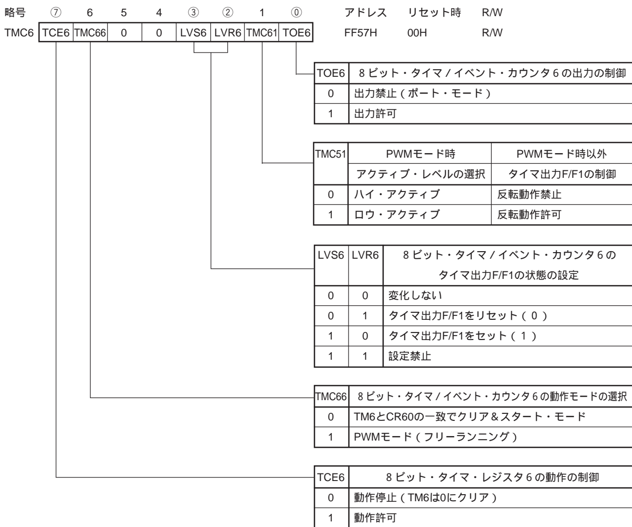
図10-6 8ビット・タイマ・モード・コントロール・レジスタ6のフォーマット
