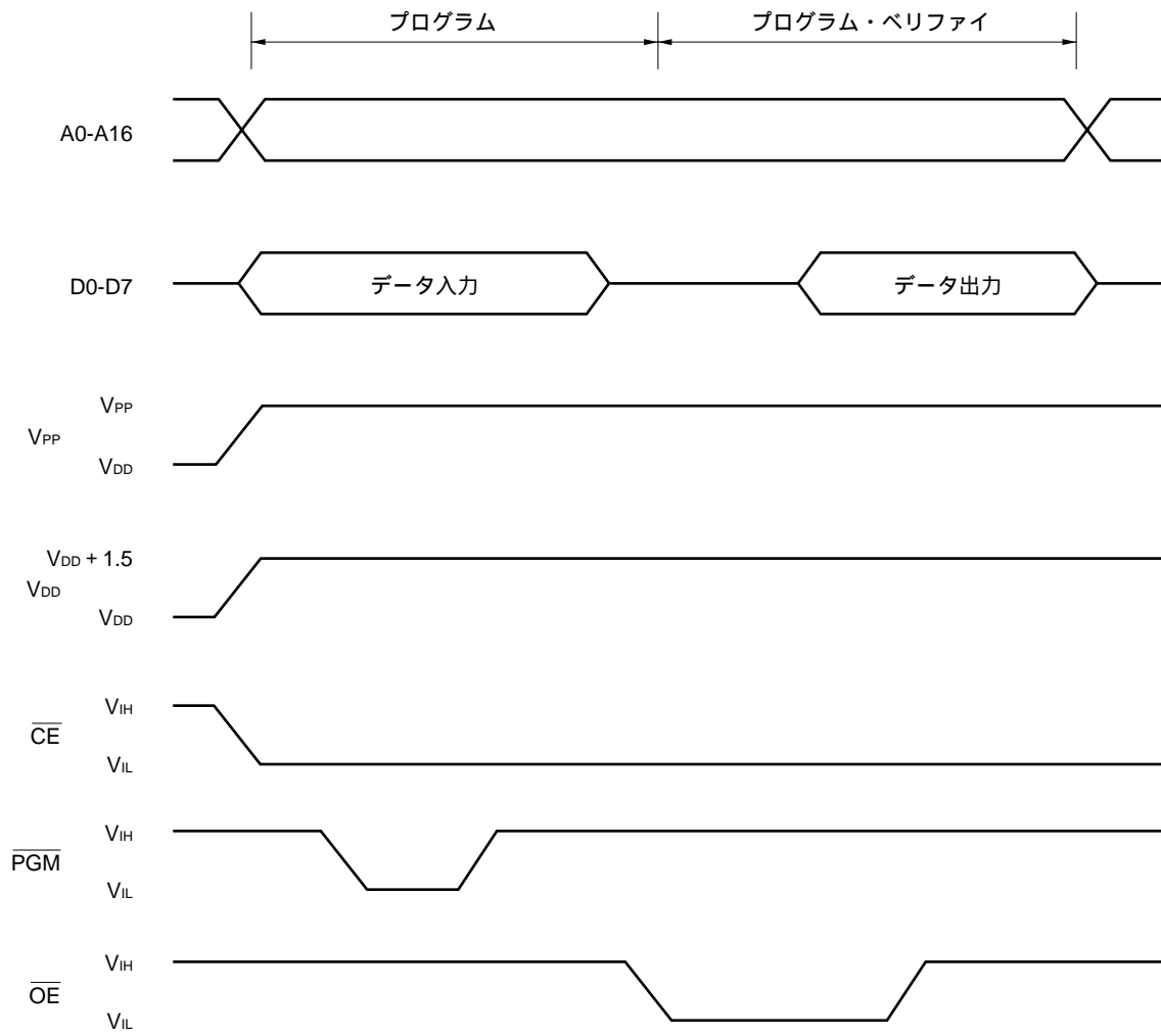
図26 - 8 バイト・プログラム・モード・タイミング
