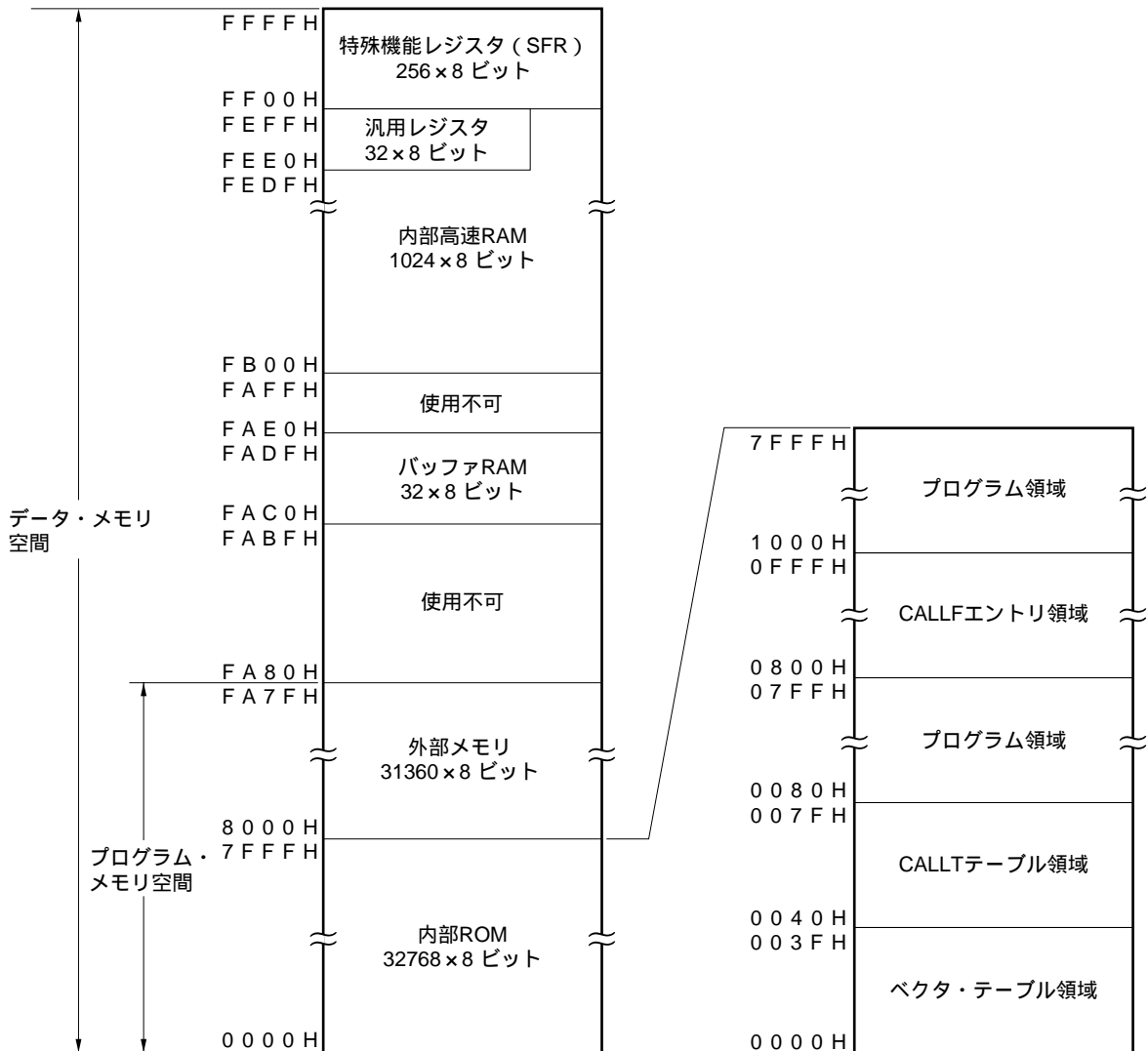
図5 - 1 メモリ・マップ (μPD78074B, 78074BY)
