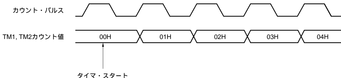
図9 - 14 8ビット・タイマ・レジスタ1, 2のスタート・タイミング
