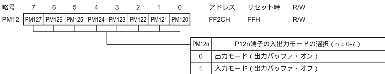
図21 - 3 ポート・モード・レジスタ12のフォーマット
