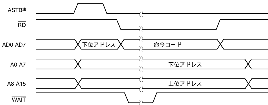
( c ) 外部ウェイト ( PW1, PW0 = 1, 1 ) 設定時
