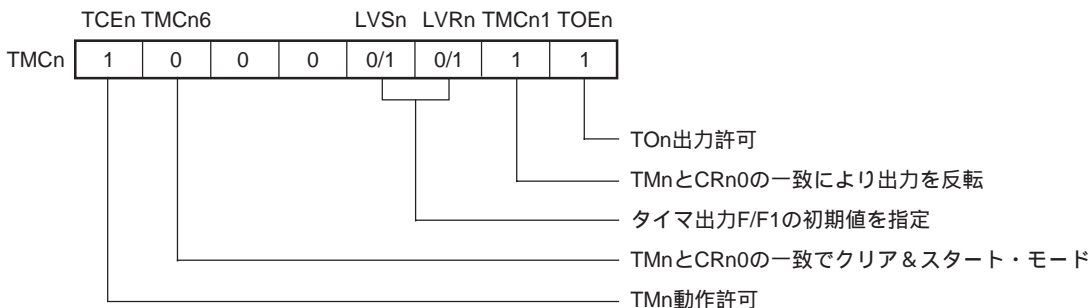
図10 - 12 方形波出力動作時の8ビット・タイマ・モード・コントロール・レジスタの設定内容
