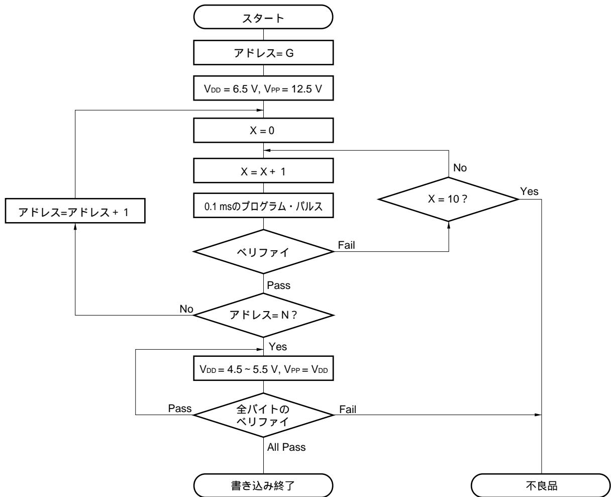
図26 - 7 バイト・プログラム・モード・フロー・チャート
