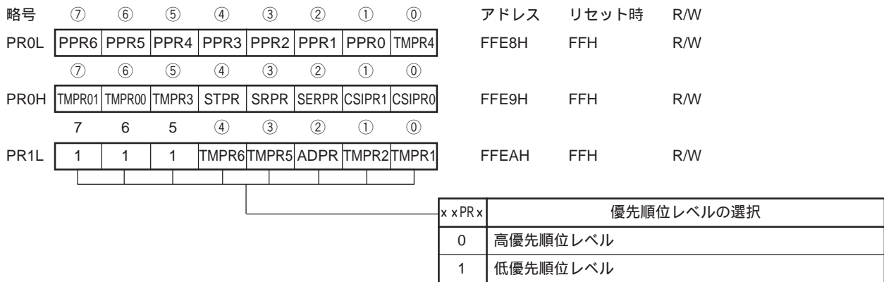
図22 - 4 優先順位指定フラグ・レジスタのフォーマット
