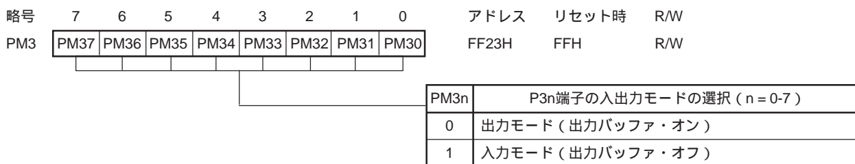
図9-7 ポート・モード・レジスタ3のフォーマット
