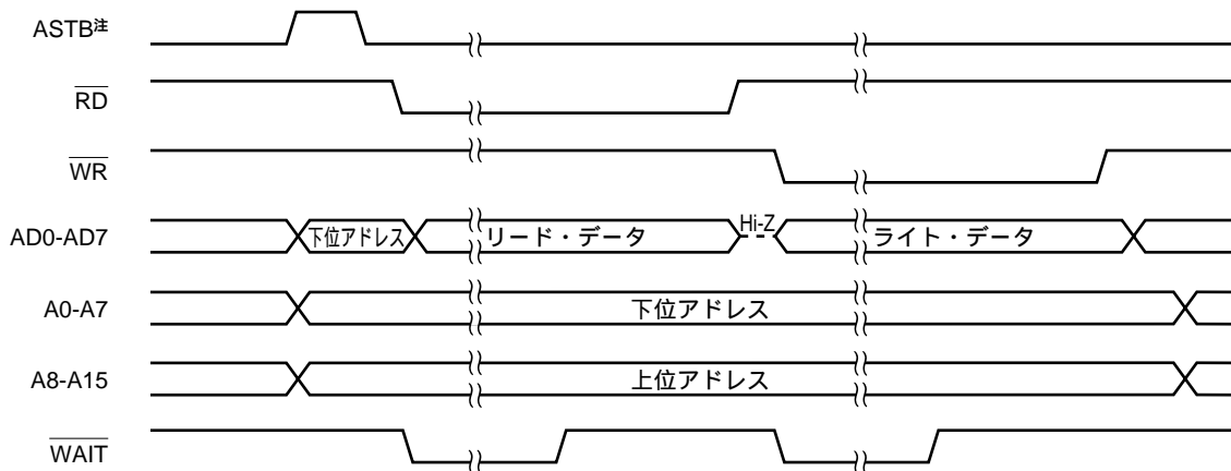
( c ) 外部ウェイト (PW1, PW0 = 1, 1) 設定時
