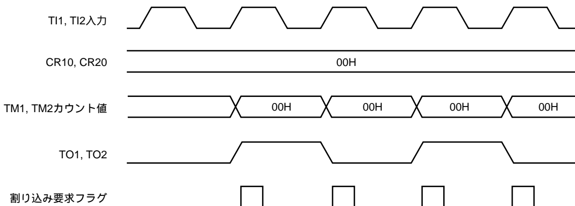
図9 - 15 外部イベント・カウンタとして動作時のタイミング
