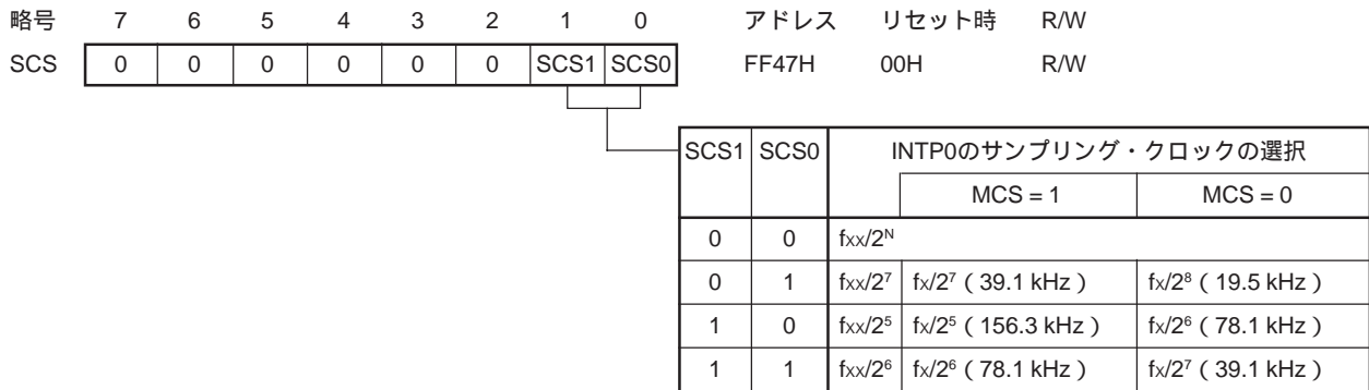
図22 - 7 サンプルング・クロック選択レジスタのフォーマット
