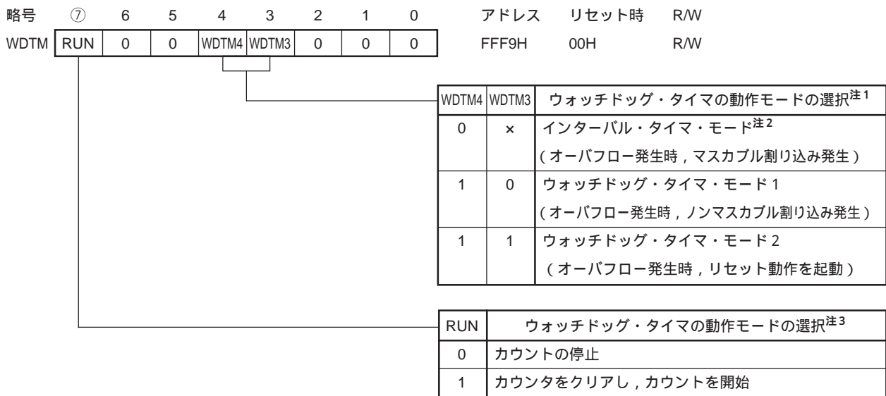
図12-3 ウォッチドッグ・タイマ・モード・レジスタのフォーマット
