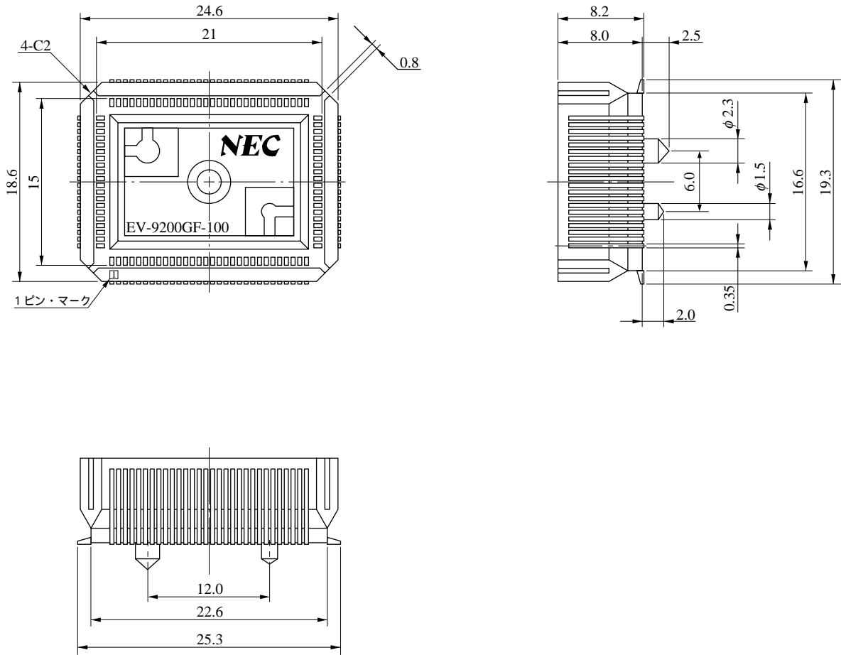
図B - 3 EV-9200GF-100 外形図 (参考) (単位: mm)
