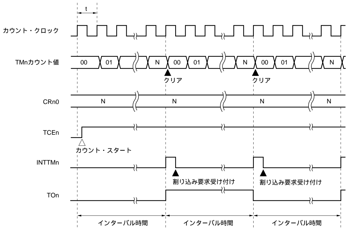
図10 - 9 インターバル・タイマ動作のタイミング
