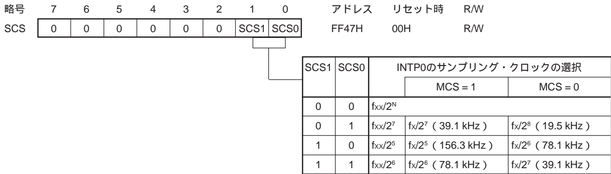
図8-9 サンプルング・クロック選択レジスタのフォーマット
