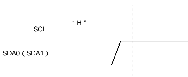
図18 - 19 ストップ・コンディション
