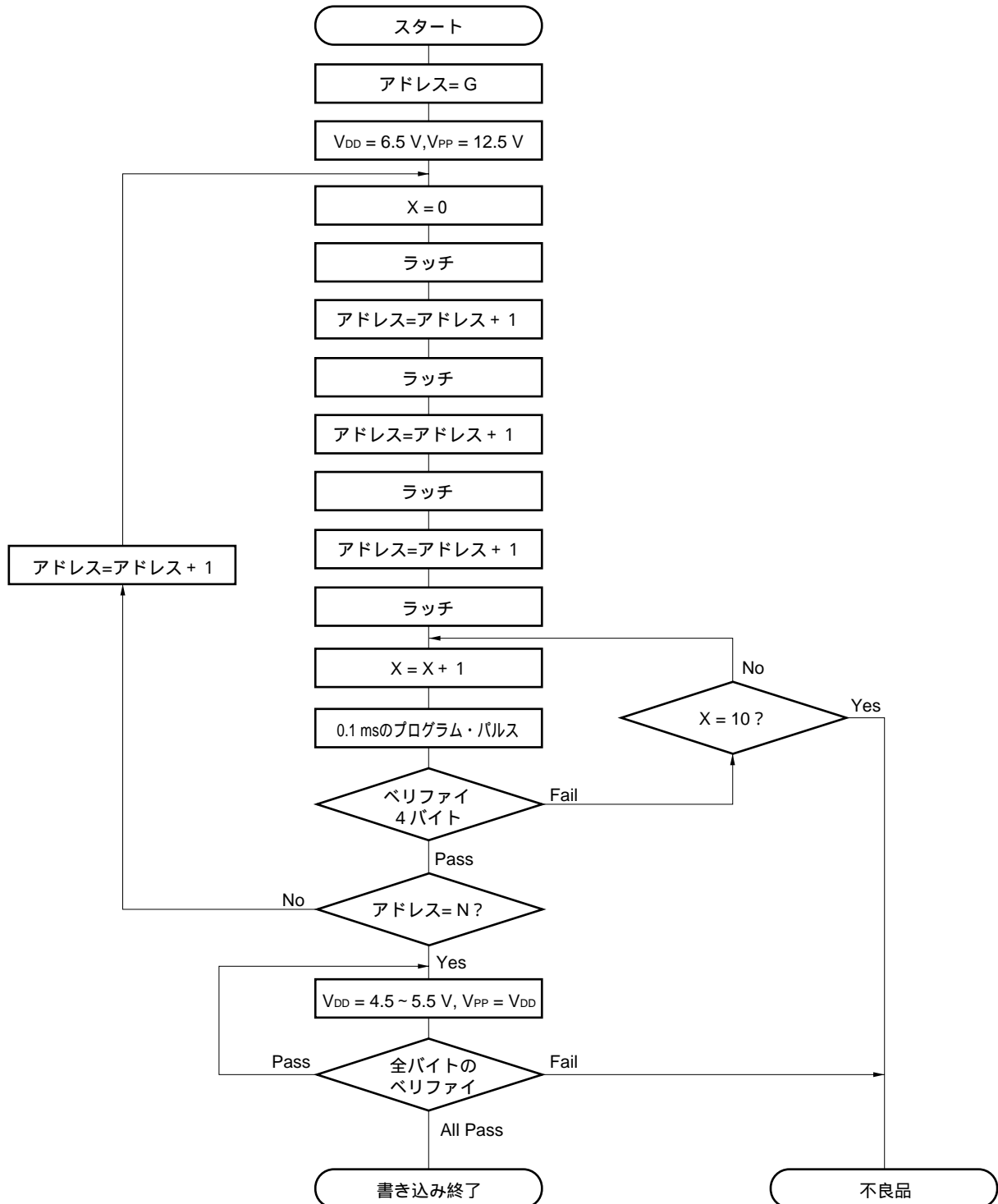
図26 - 5 ページ・プログラム・モード・フロー・チャート
