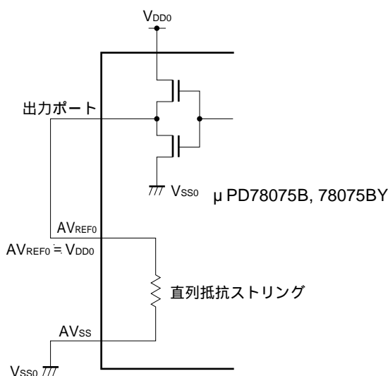
図15-9 スタンバイ・モード時の消費電流を低減させる方法例
