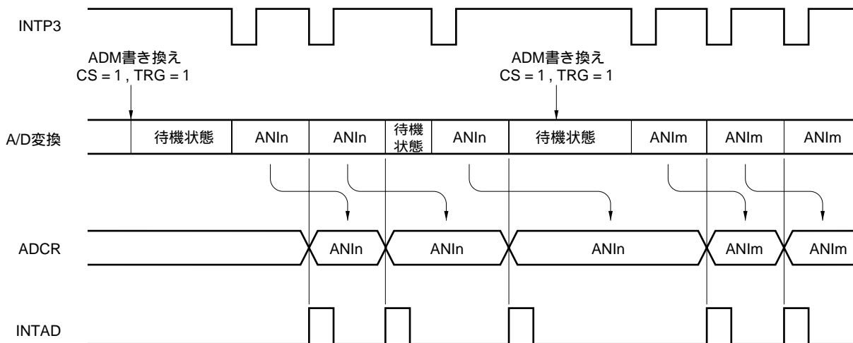
図15 - 7 ハードウェア・スタートによるA/D変換動作
