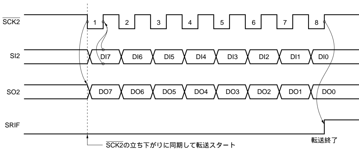
図20 - 12 3線式シリアルI/Oモードのタイミング
