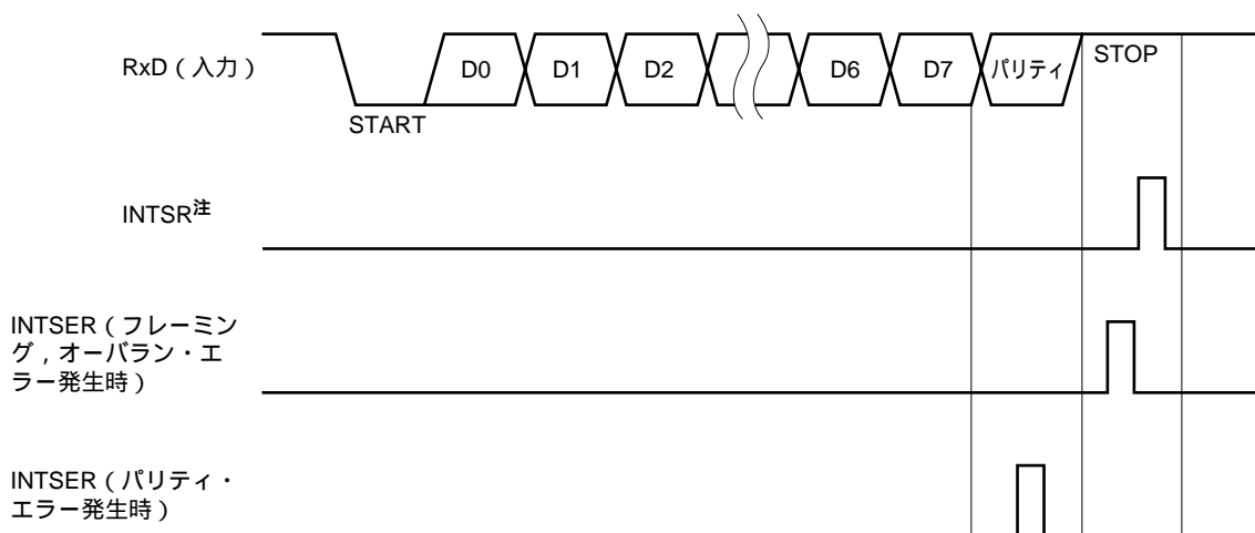
図20 - 10 受信エラー・タイミング
