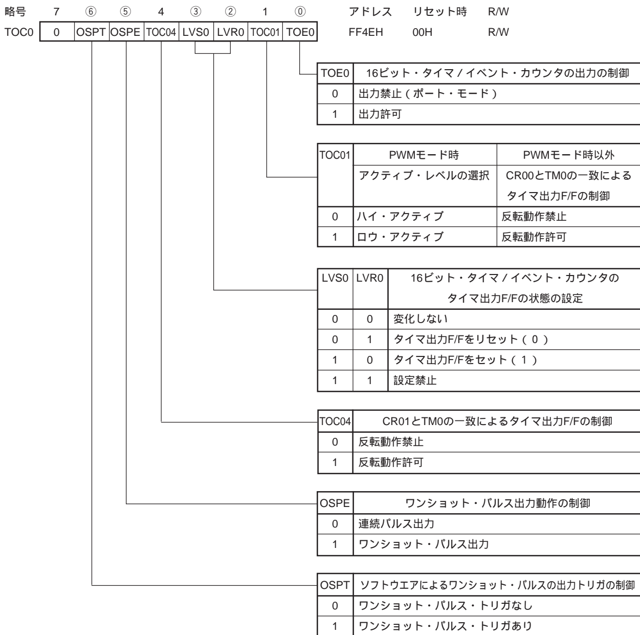
図8 - 6 16ビット・タイマ出力コントロール・レジスタのフォーマット
