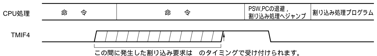
図22 - 11 ノンマスクابل割り込み要求の受け付けタイミング
