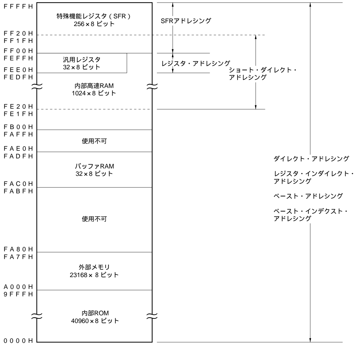
図5 - 4 データ・メモリのアドレッシング (μPD78075B, 78075BY)
