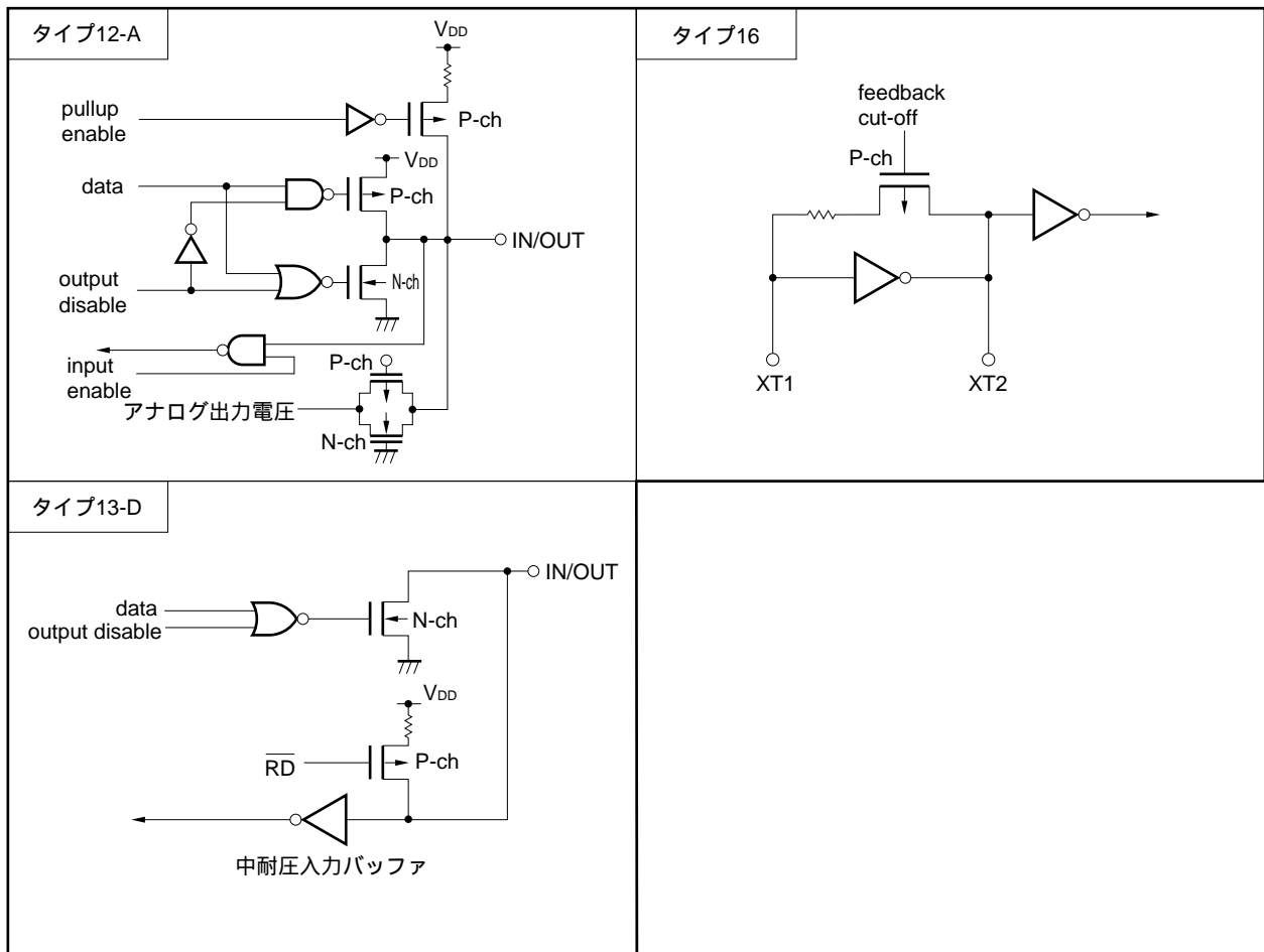
図26 - 1 端子の入出力回路一覧 (2/2)
