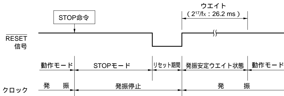
図24 - 5 STOPモードの \overline{\text{RESET}} 入力による解除
