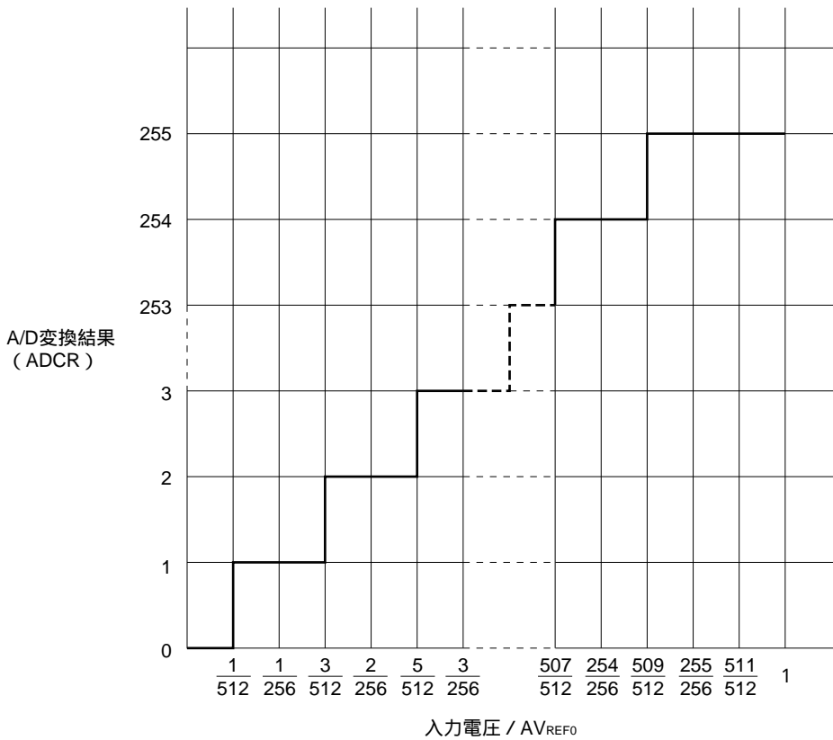
図15 - 6 アナログ入力電圧とA/D変換結果の関係
