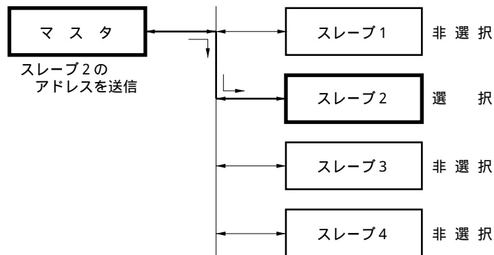
図17-15 アドレスによるスレーブの選択
