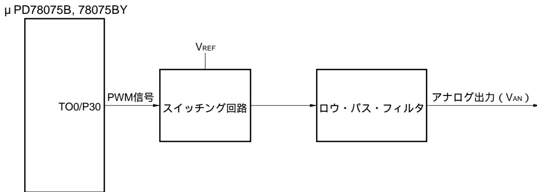
図8 - 14 PWM出力によるD/Aコンバータ構成例
