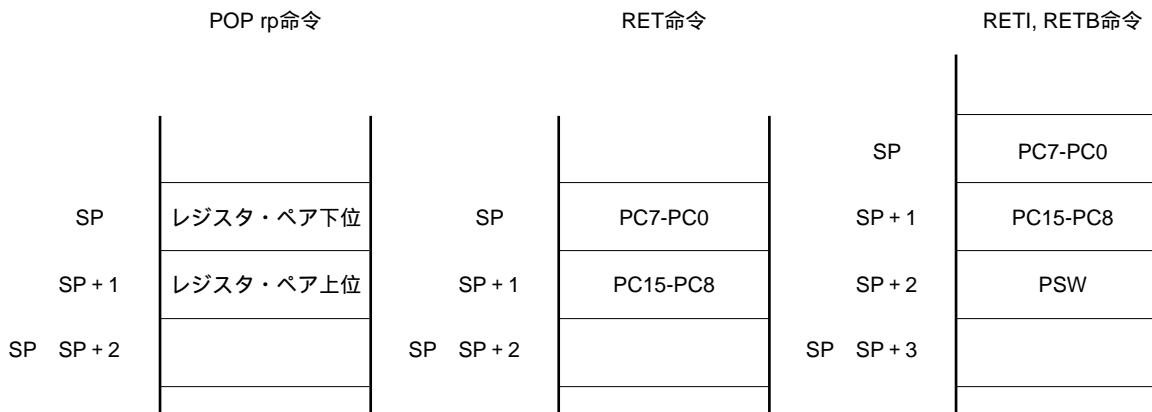
図5 - 9 スタック・メモリから復帰されるデータ
