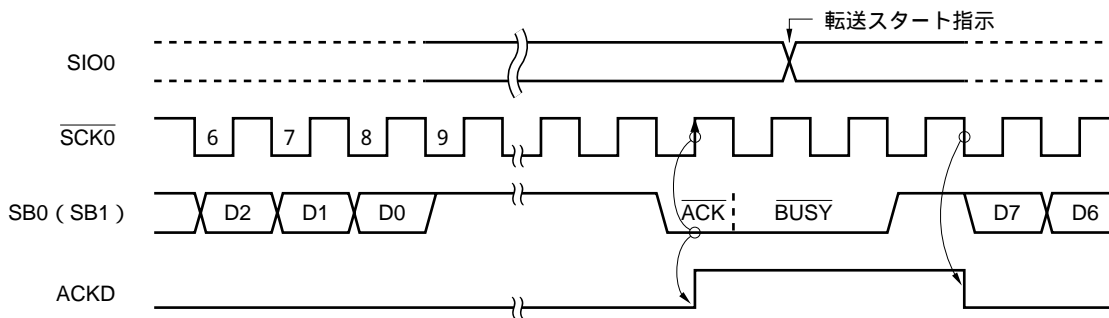
図17-25 BSYEの動作
