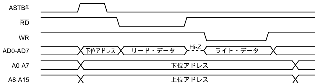
( b ) ウェイトあり (PW1, PW0 = 0, 1) 設定時
