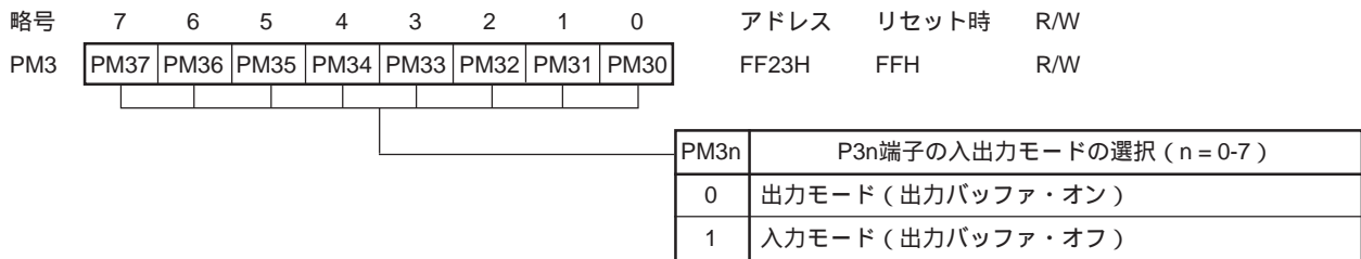
図13 - 4 ポート・モード・レジスタ3のフォーマット
