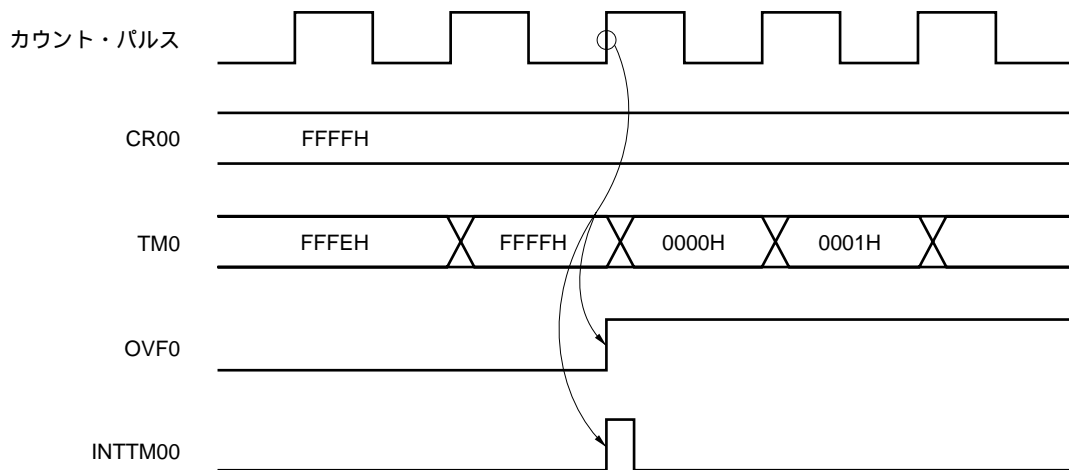
図8 - 38 OVF0フラグの動作のタイミング
