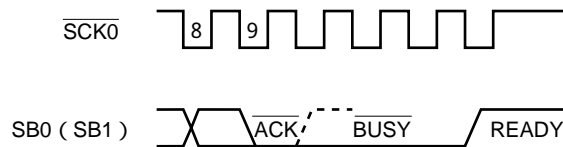
図17 - 19 ビジィ信号, レディ信号
