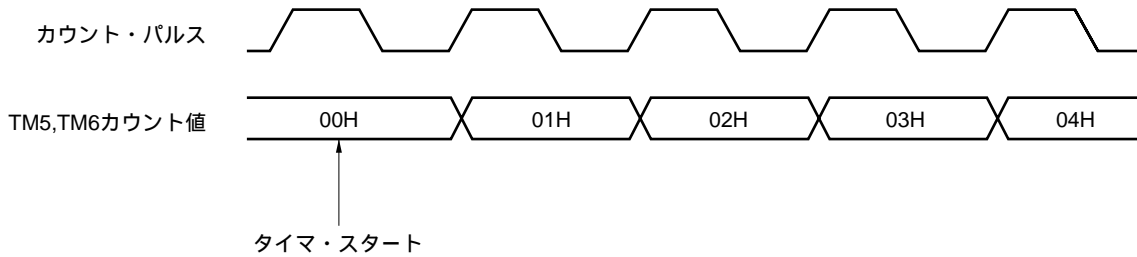
図10-19 8ビット・タイマ・レジスタ5, 6のスタート・タイミング
