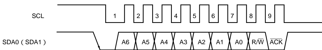
図18 - 18 アクノリッジ信号
