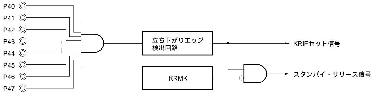
図6 - 11 立ち下がりエッジ検出回路のブロック図
