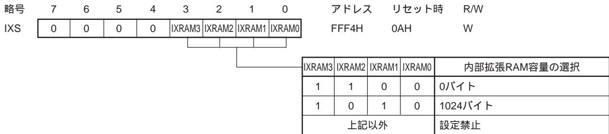
図26 - 4 内部拡張RAMサイズ切り替えレジスタのフォーマット
