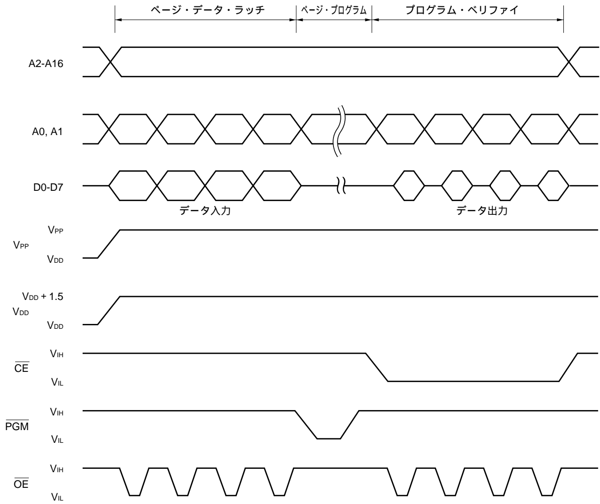
図26 - 6 ページ・プログラム・モード・タイミング
