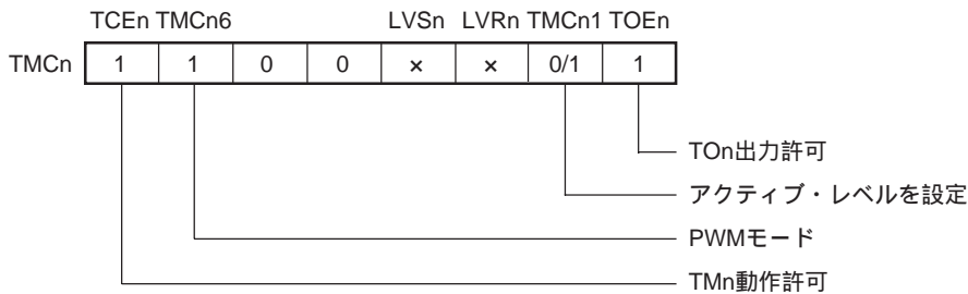
図10 - 14 PWM出力動作時の8ビット・タイマ・モード・コントロール・レジスタの設定内容
