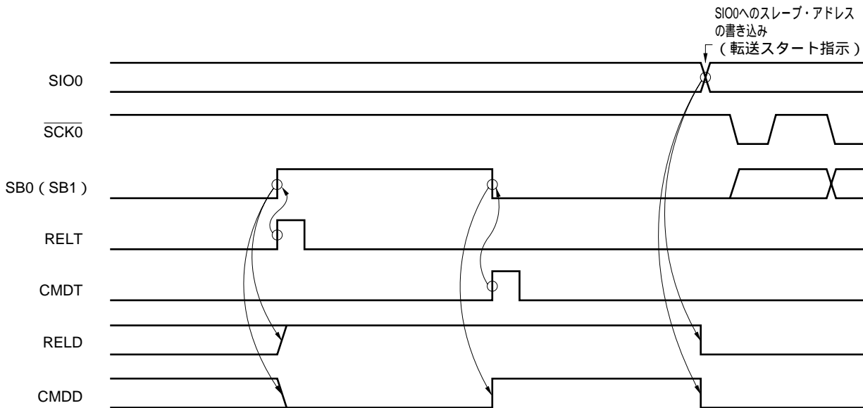
図17 - 21 RELD, CMDDの動作 (スレーブ)
