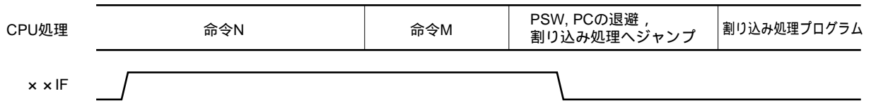
図22 - 17 割り込み要求の保留
