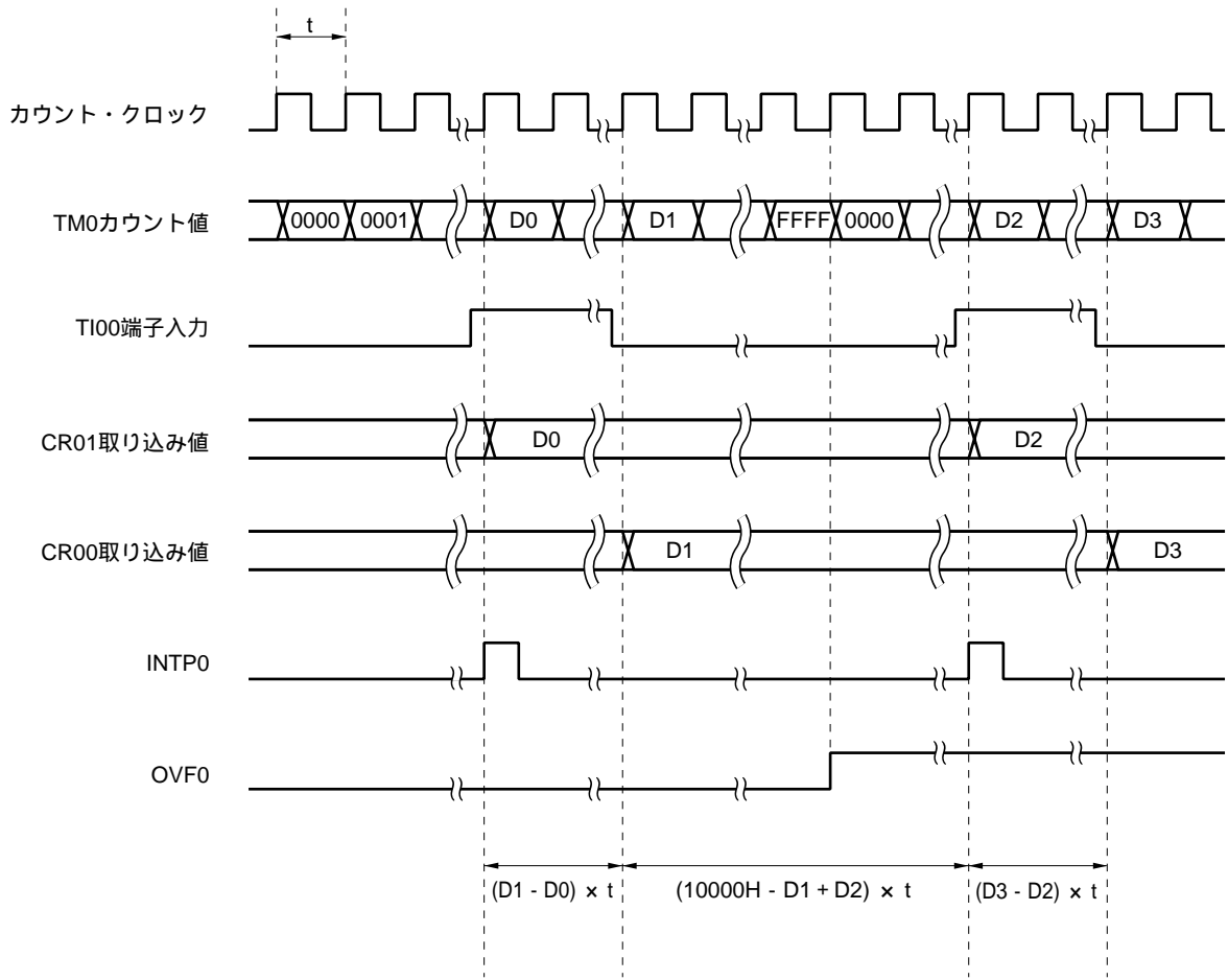
図8 - 23 フリーランニング・カウンタとキャプチャ・レジスタ2本によるパルス幅測定動作のタイミング (立ち上がりエッジ指定時)
