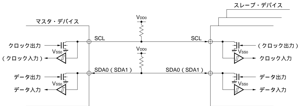
図18 - 21 端子構成図
