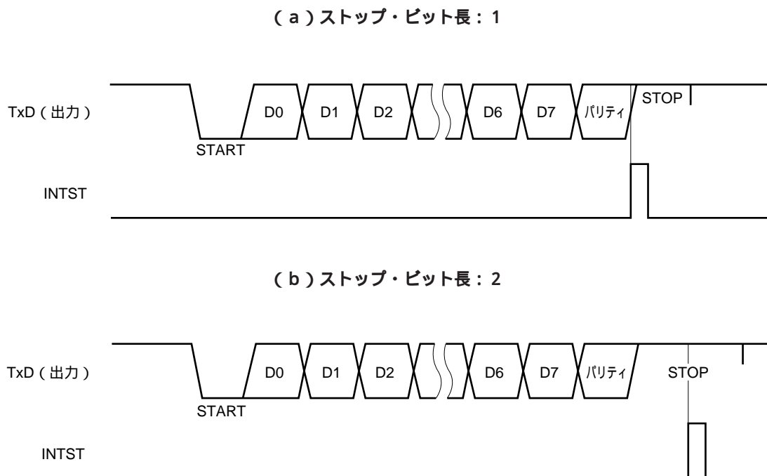
図20 - 8 アシクロナス・シリアル・インタフェース送信完了割り込み要求タイミング
