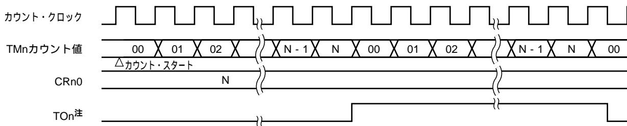
図10 - 13 方形波出力動作のタイミング
