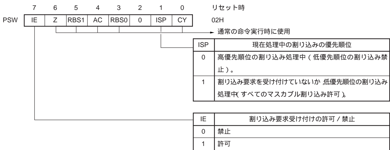
図22 - 9 プログラム・ステータス・ワードの構成
