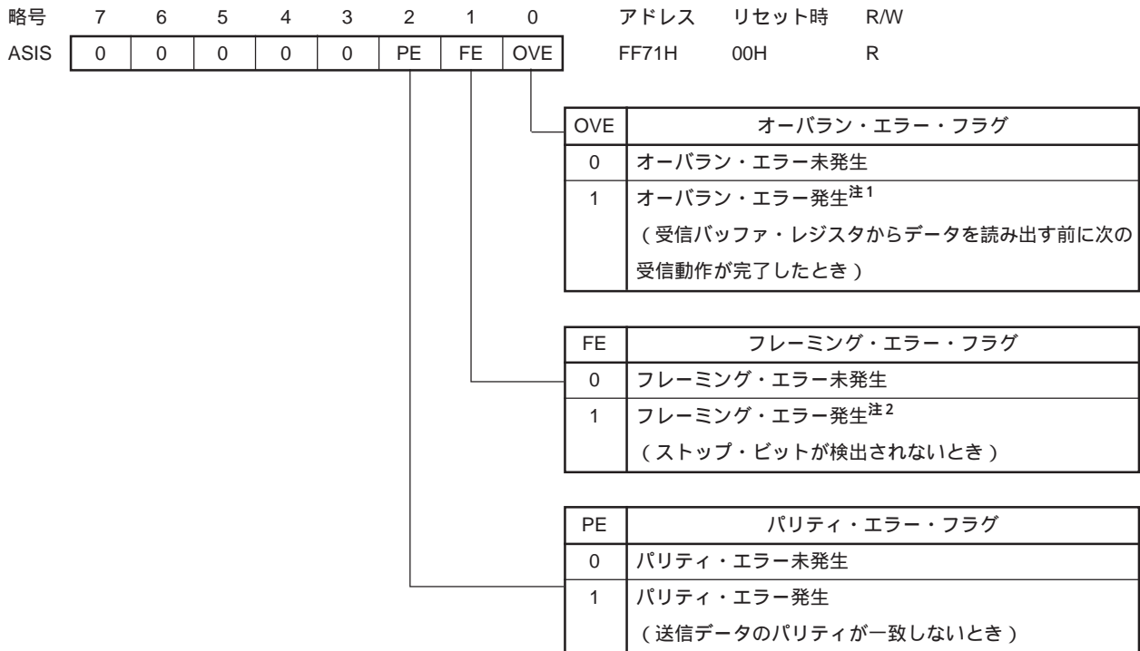
図20 - 5 アシクロナス・シリアル・インタフェース・ステータス・レジスタのフォーマット
