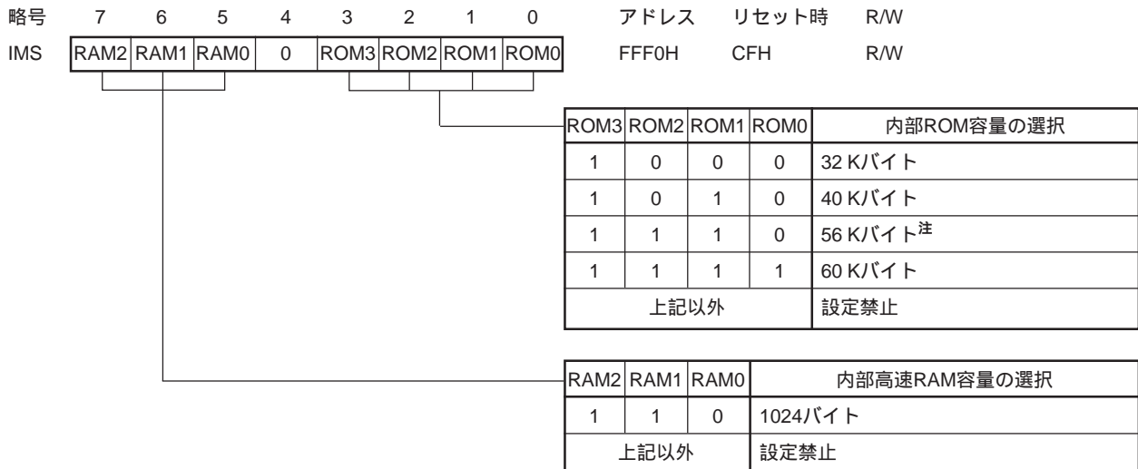
図26 - 3 メモリ・サイズ切り替えレジスタのフォーマット
