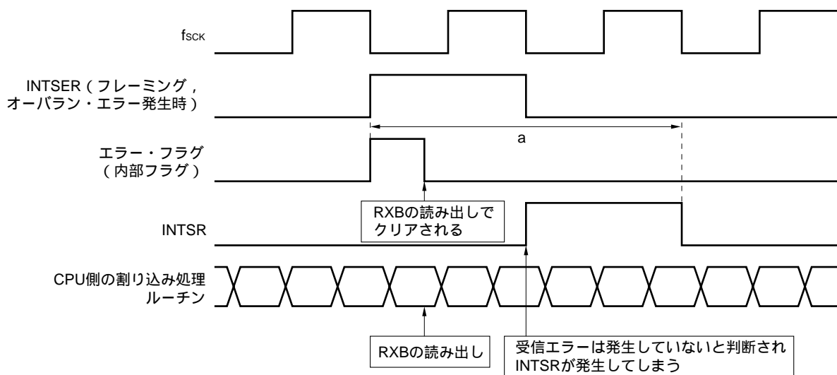
図20-14 受信完了割り込みの発生タイミング (ISRM = 1 のとき)
