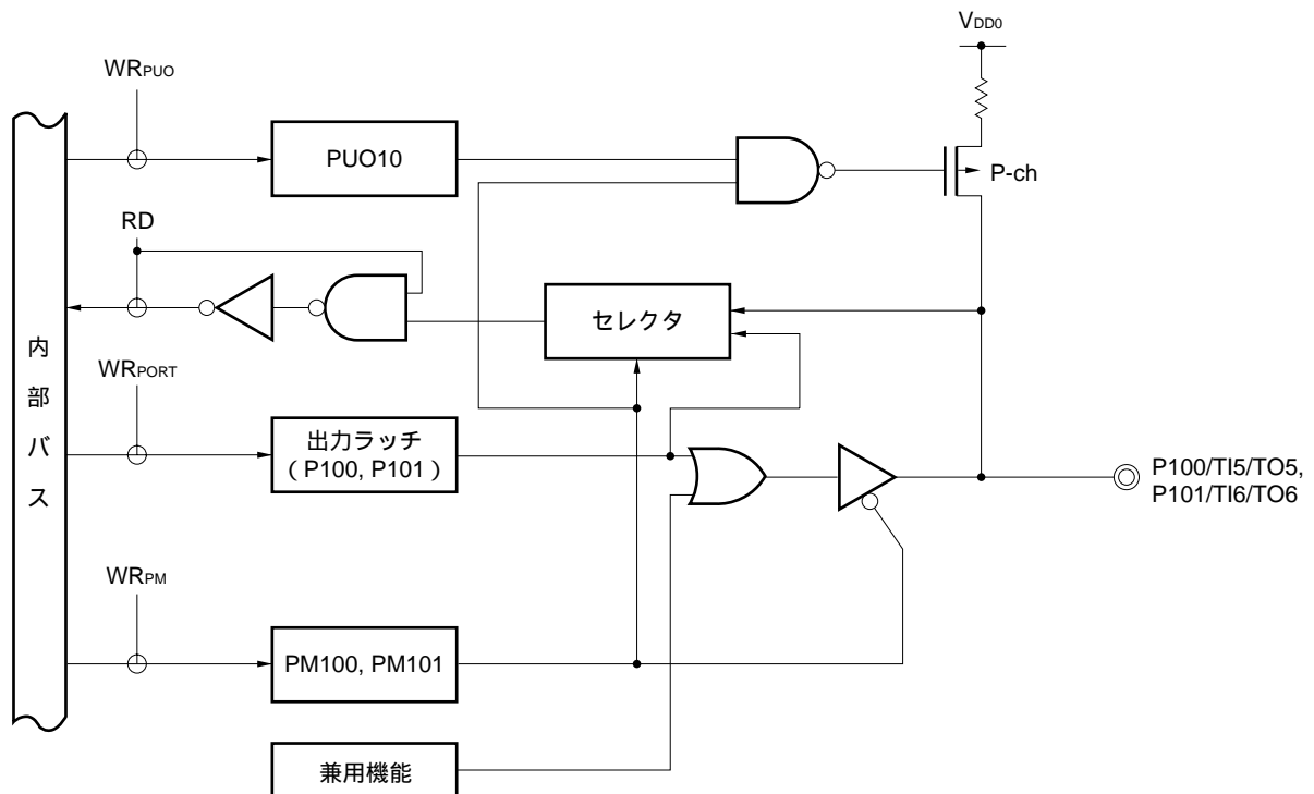
図6-20 P100, P101のブロック図
