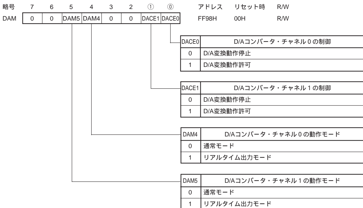
図16 - 2 D/Aコンバータ・モード・レジスタのフォーマット
