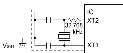
(a) クリスタル発振
