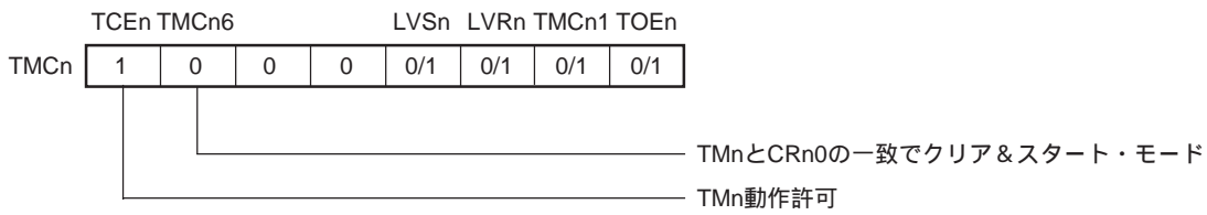
図10 - 8 インターバル・タイマ動作時の8ビット・タイマ・モード・コントロール・レジスタの設定内容
