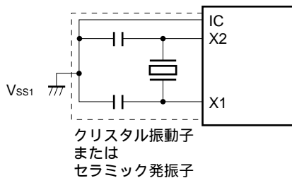
(a) クリスタル, セラミック発振
