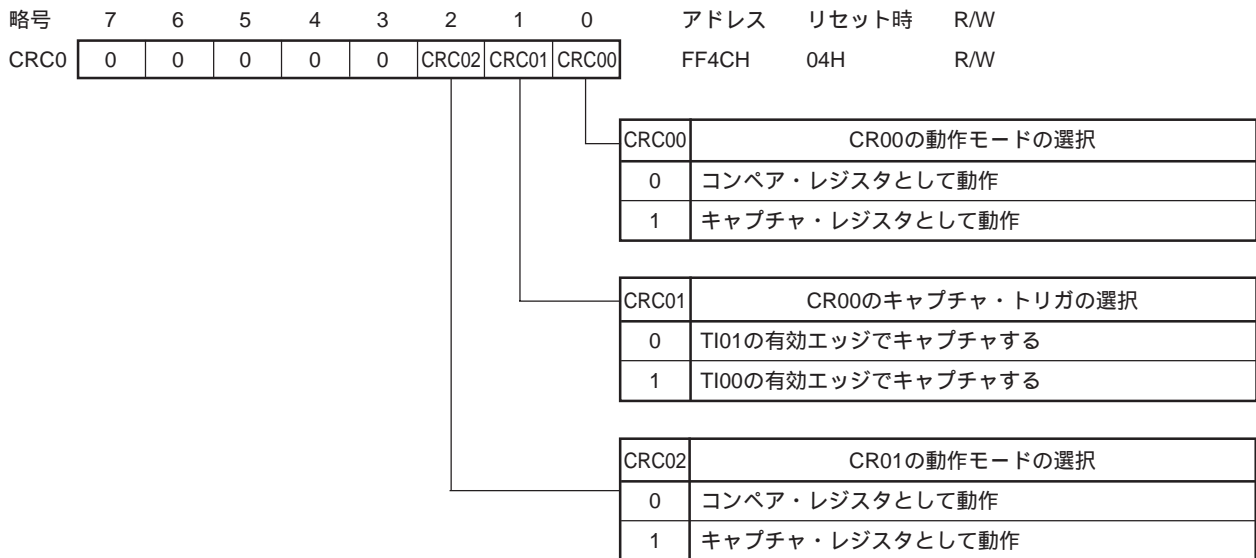
図8-5 キャプチャ/コンペア・コントロール・レジスタ0のフォーマット
