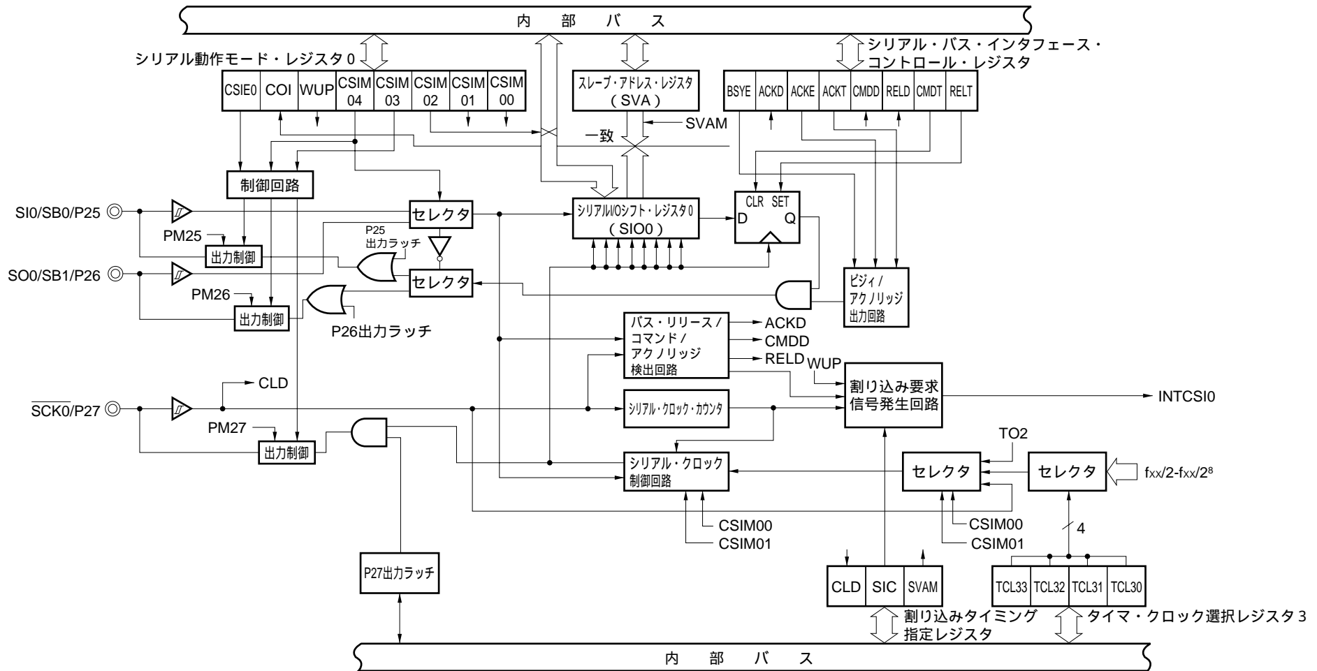
図17-2 シリアル・インタフェース・チャンネル0のブロック図
