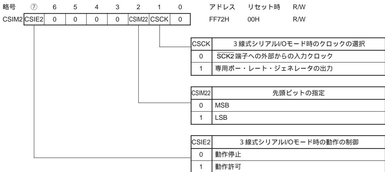
図20 - 3 シリアル動作モード・レジスタ2のフォーマット
