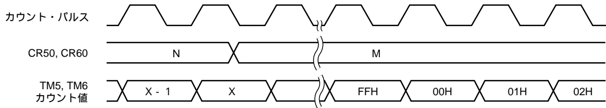
図10-21 タイマ・カウント動作中のコンペア・レジスタの変更後のタイミング
