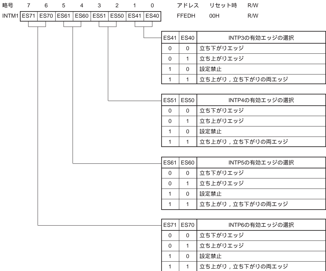
図22 - 6 外部割り込みモード・レジスタ1のフォーマット
