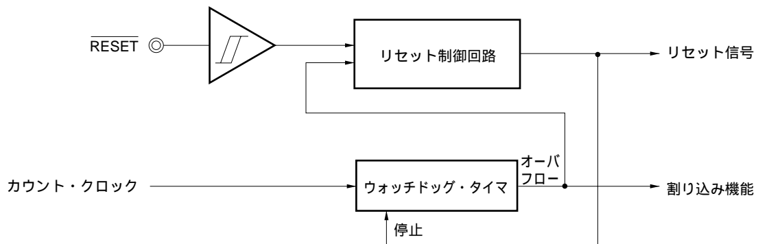
図25 - 1 リセット機能のブロック図
