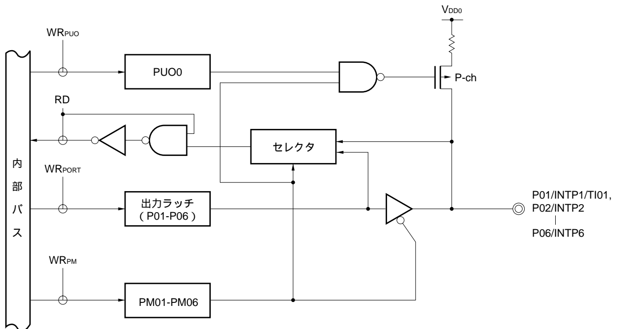
図6-3 P01-P06のブロック図
