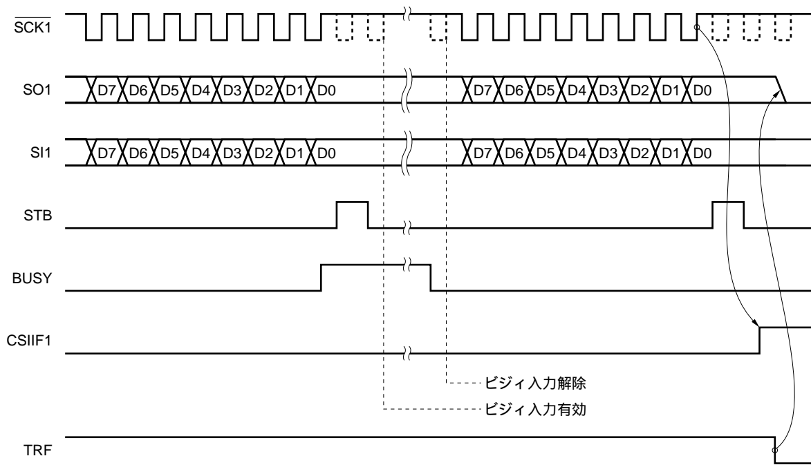
図19 - 21 ビジィ&ストローブ制御オプションを使用したときの動作タイミング(BUSY0 = 0のとき)
