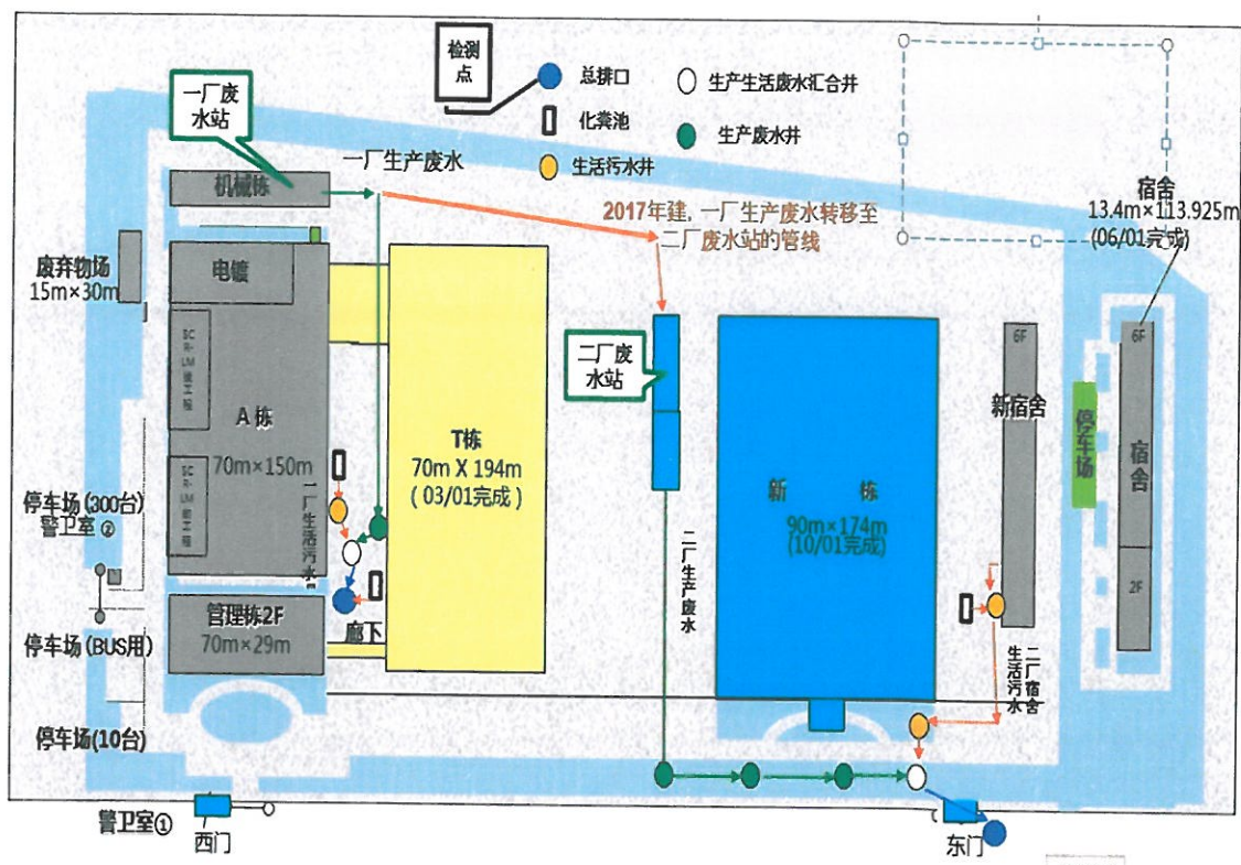
图 4-4 污水管线图
