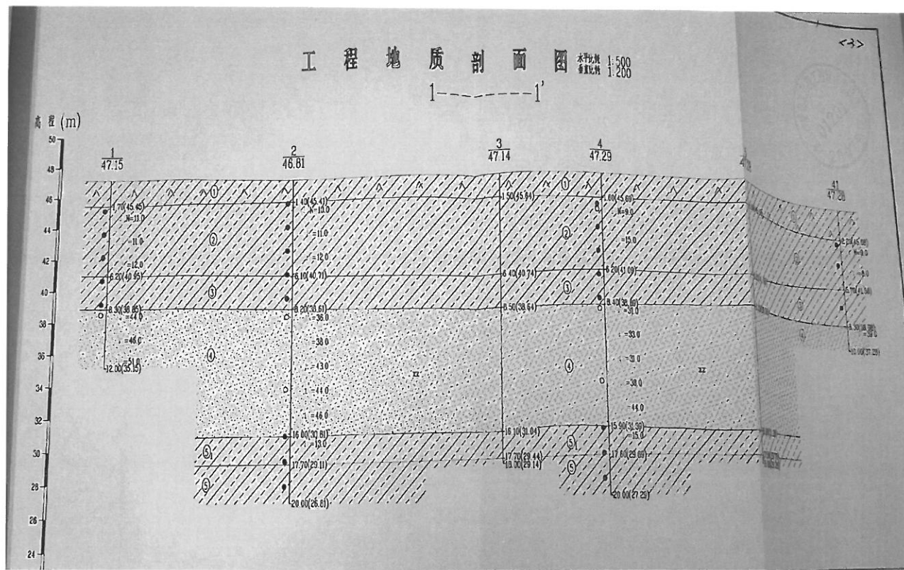
图 8 工程地质剖面图
