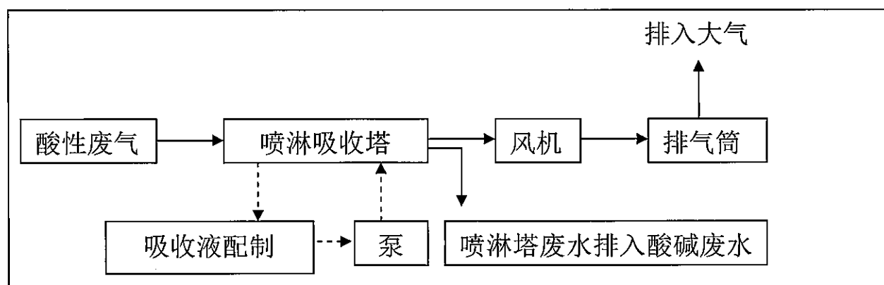
图 2 废气处理工艺流程图
