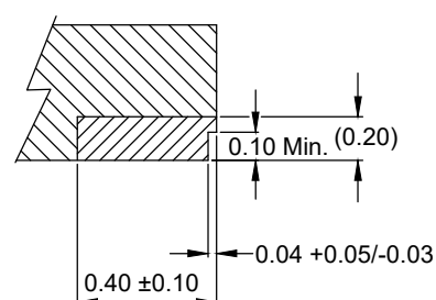
Section : A-A Scale : NTS
