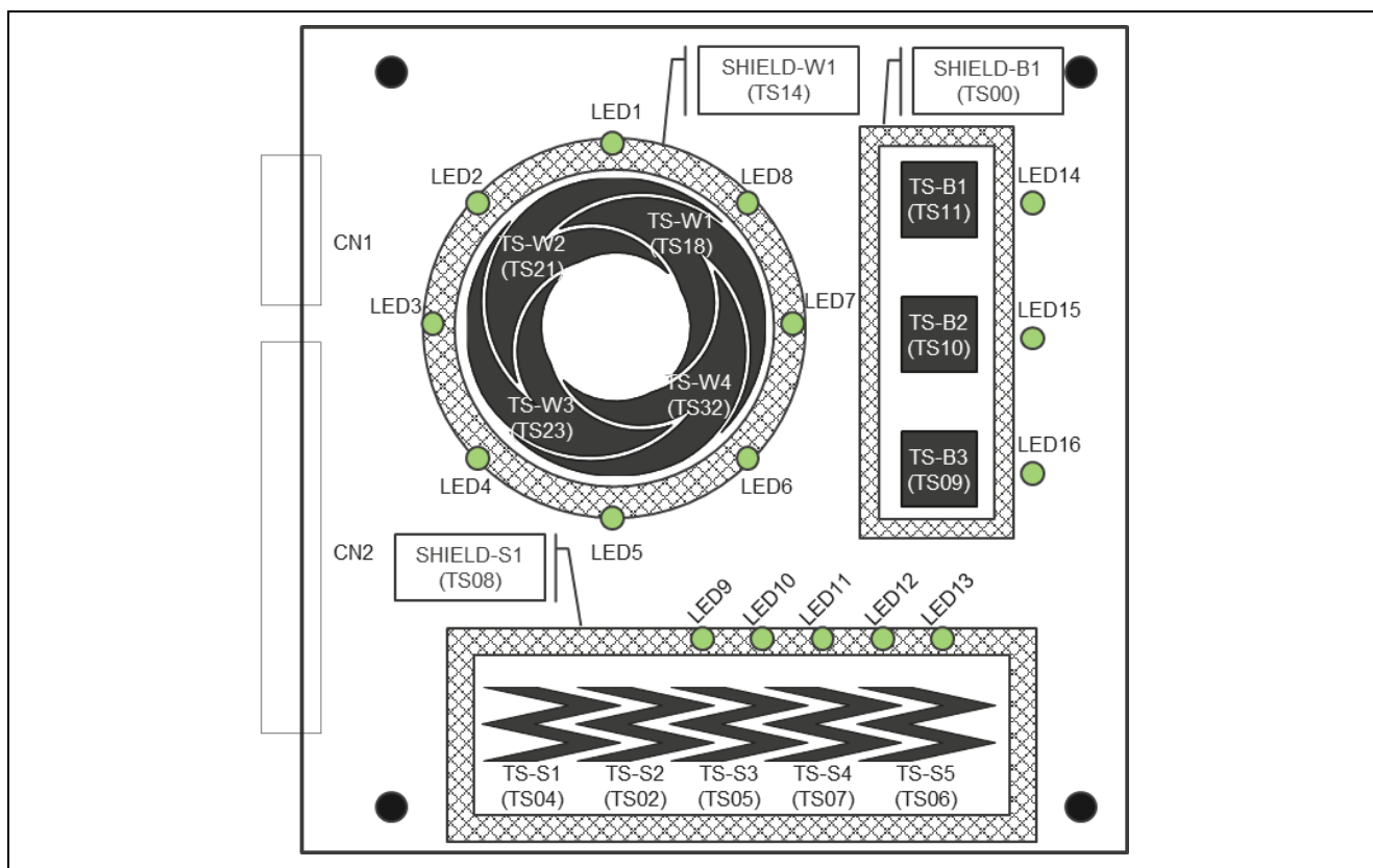
図.1 タッチ電極と TS 端子の割り当て
