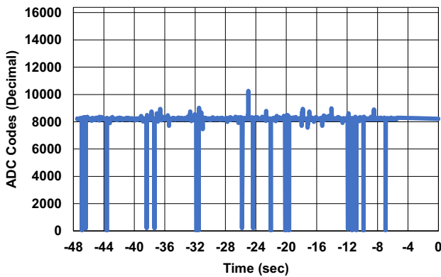
Figure 14. SET at AV CC = 4.5V, f S = 750kps, and LET = 86
