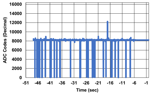
Figure 15. SET at AV CC = 4.5V, f S = 1000kps, and LET = 86
