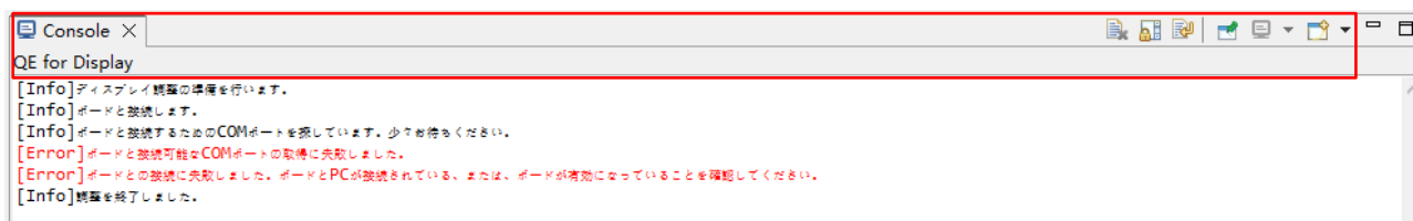
図 3-5 Console ビュー
