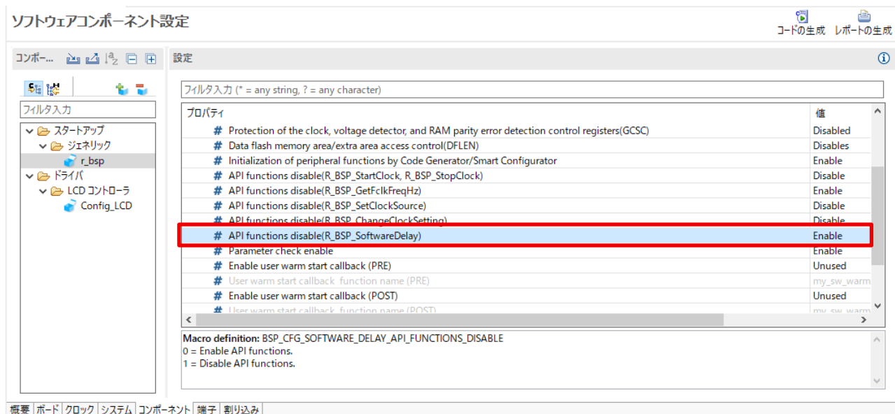
図 3-6 R_BSP_SoftwareDelay 関数の有効化
