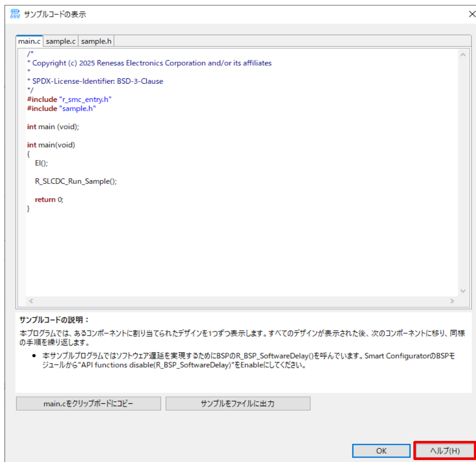
図 3-5 サンプルコードの表示ダイアログ上の「ヘルプ(H)」ボタン
