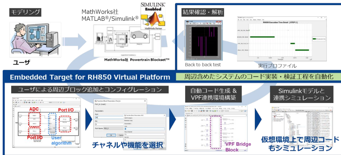
図 1 全体イメージ図 (RH850)
