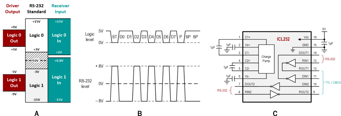
图 2：RS-232 信号电平（A），从逻辑转换为总线信号（B），带有集成电荷泵的 RS-232 收发器（C）
