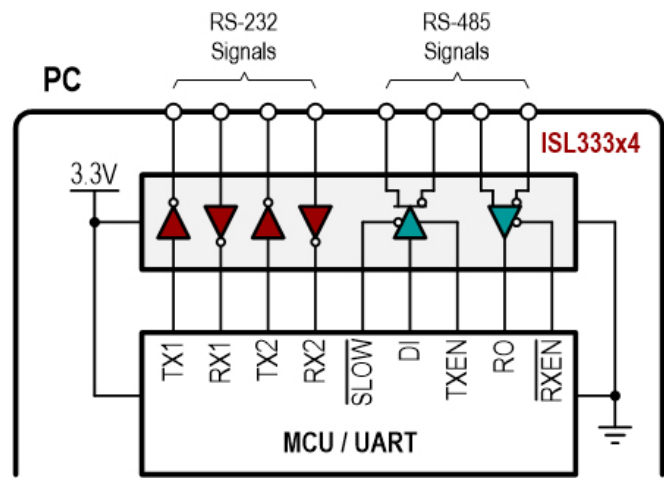
图 7：通过 RS-232 至 RS-485 转换器连网多个 RS-232 设备
