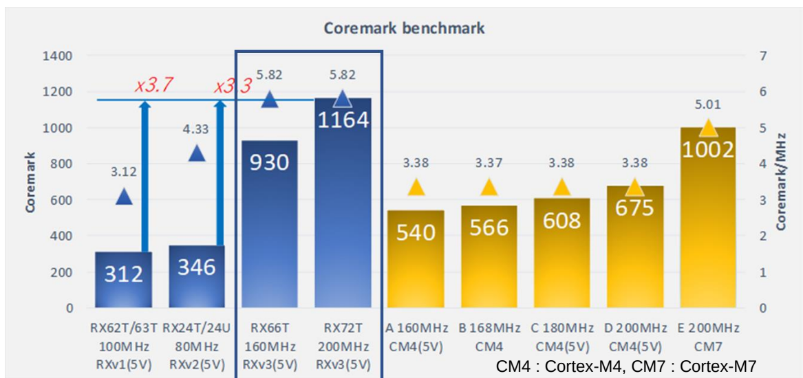
図 7. コアマーク ベンチマーク比較
