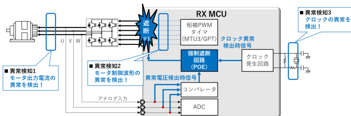
図 6. 三相相補 PWM 出力保護機能
