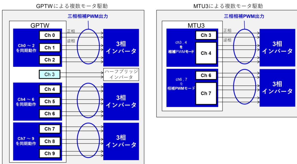
図 2. 三相相補 PWM タイマ本数
