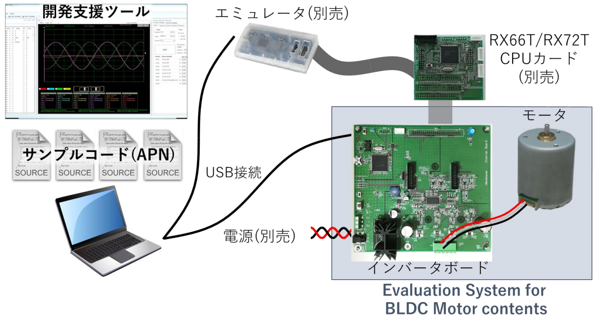
図 12. Evaluation System for BLDC Motor の構成
