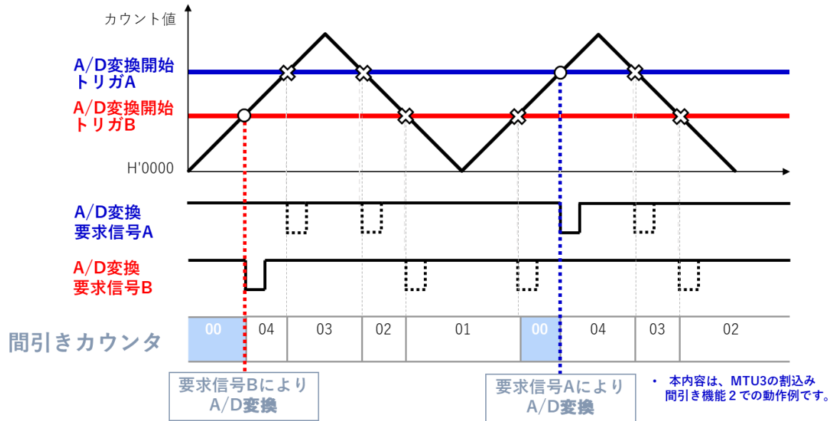
図 5. 三相相補 PWM タイマの A/D 変換間引き機能
