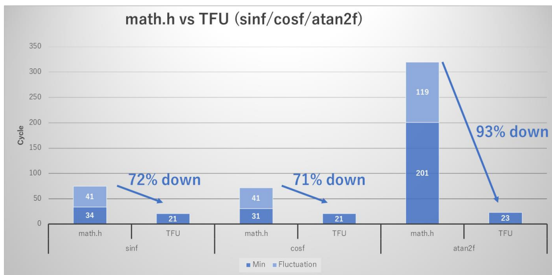
図 8. TFU の効果 math.h vs TFU
