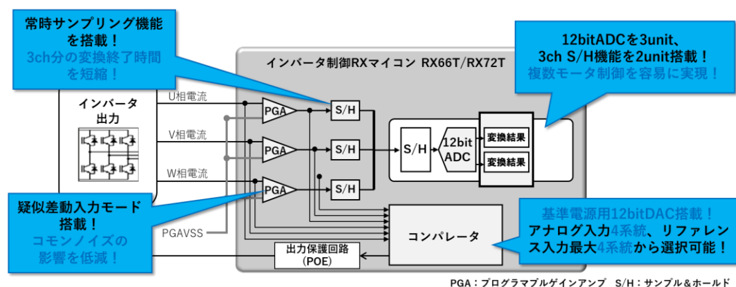
図 10. RX66T/RX72T シリーズ搭載 A/D コンバータの特長
