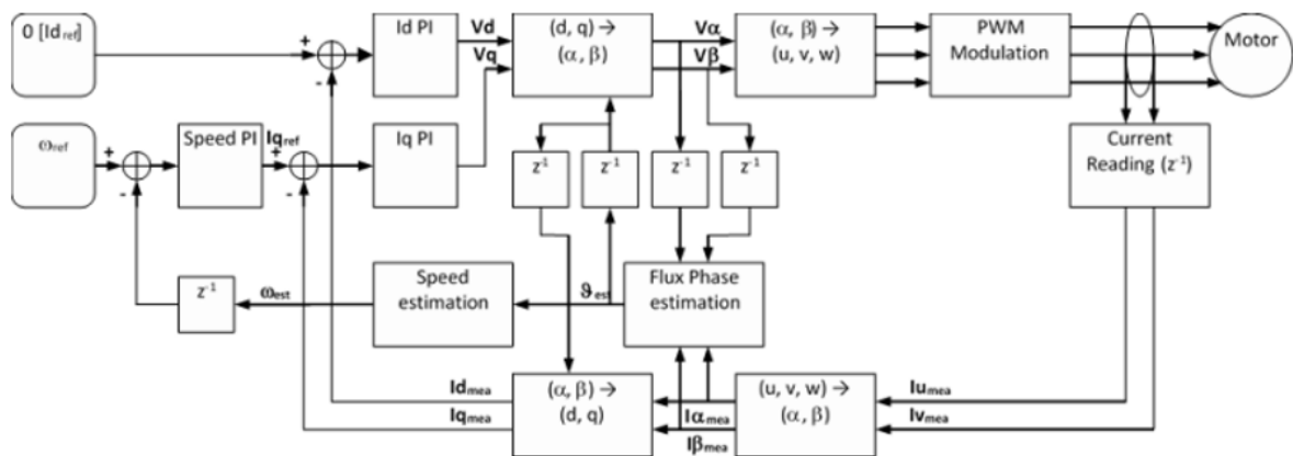
図 13. FOC アルゴリズムの構成
