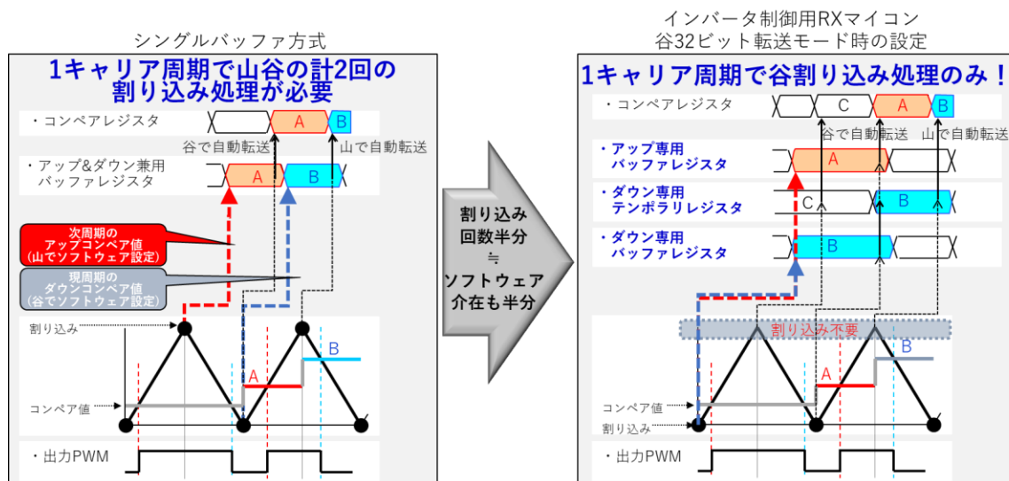
図 3. 三相相補 PWM タイマのダブルバッファ機能
