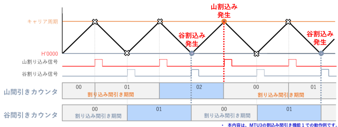
図 4. 三相相補 PWM タイマの割込み間引き機能
