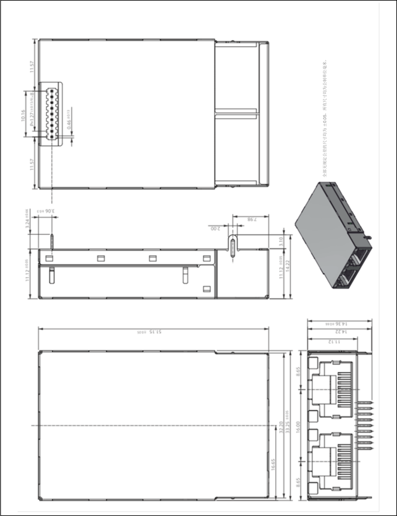
图 6.1 包装尺寸
